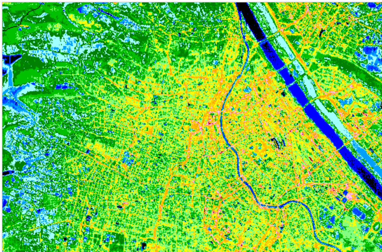
Thermalbefliegung 16.08.2001 (Morgenaufnahme)
