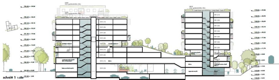
schnitt 1 1:200
