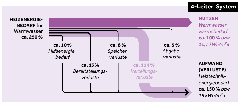
Abb. 7 Energieströme bei der Warmwasserbereitung: Größenordnungen für 2-Leiter- (oben) und 4-Leiter- (unten) System, 20 Wohnungen Quelle: ALLPLAN 15
