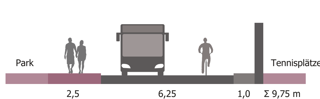
QUERSCHNITT BUSTRASSE
