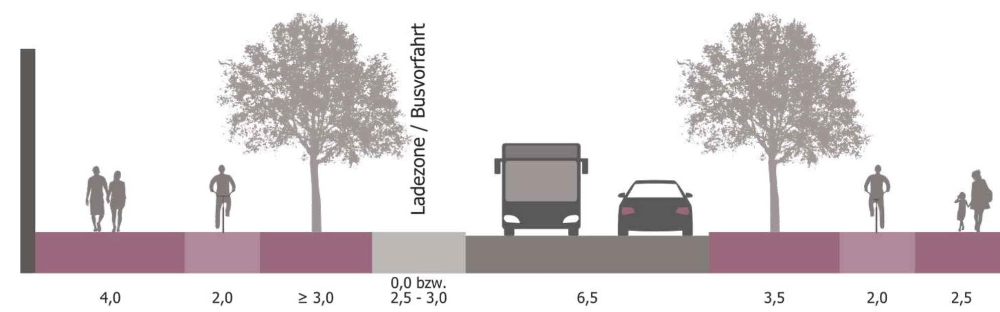
QUERSCHNITT DÖBLERHOFSTRASSE
