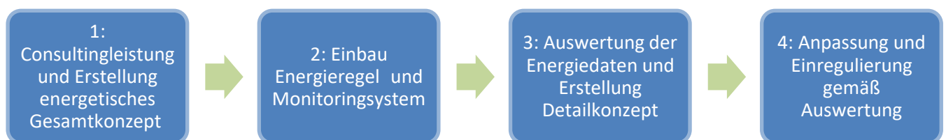
Abbildung 2: Ablaufdiagramm zur Optimierung der Energieversorgung und Erhöhung der Energieeffizienz eines Gebäudes
