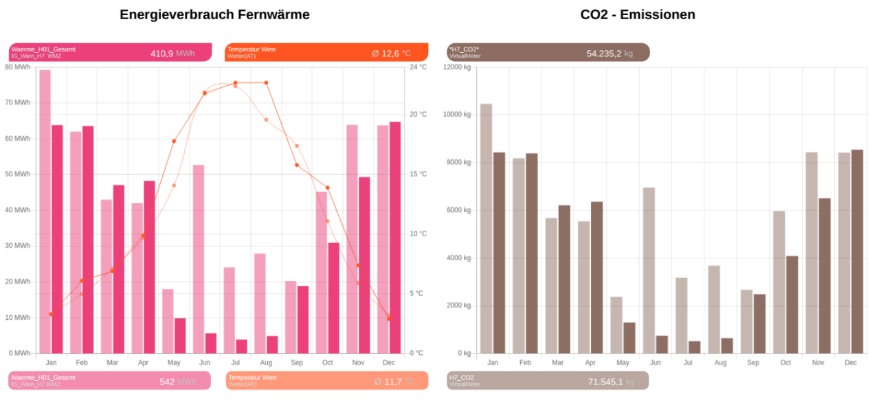
Abbildung 1: Auswertung des Energieverbrauchs eines fernwärmeversorgten Gebäudes mit verschiedenen Nutzungen
