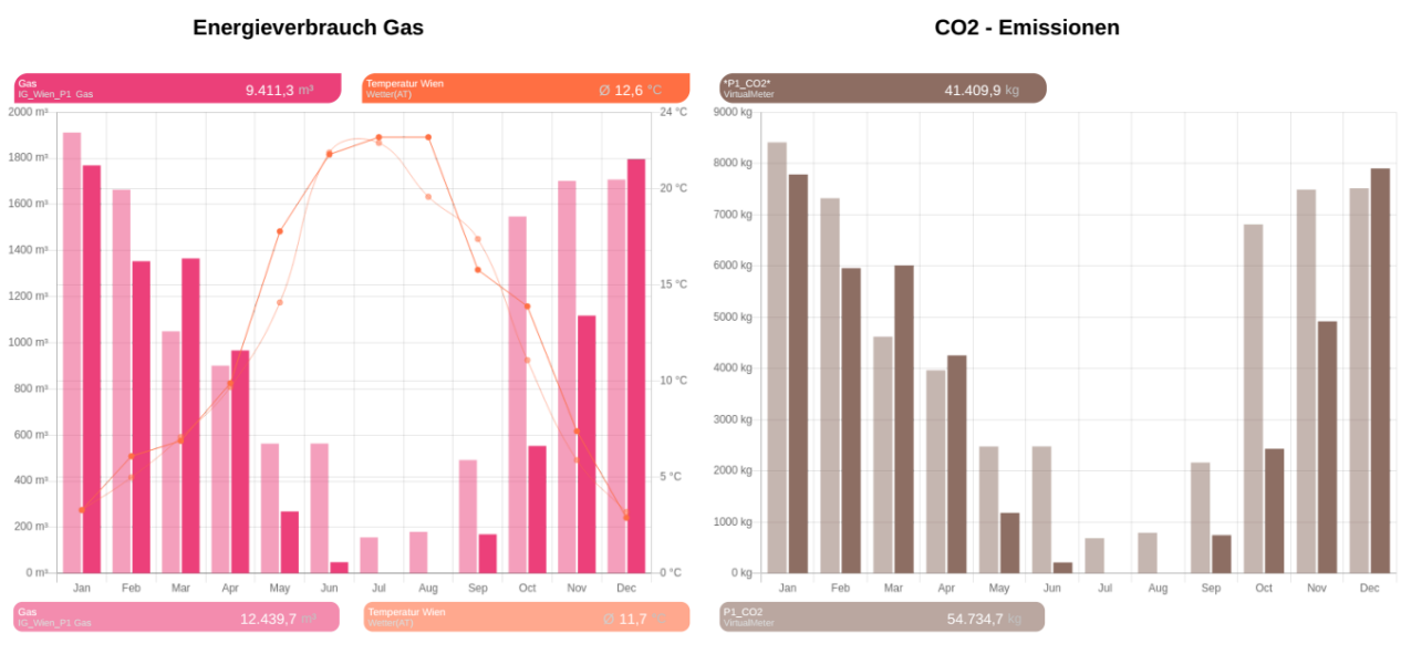
Abbildung 3: Beispiel eines Auswertungsdiagramms für ein gasversorgtes Gebäude - dargestellt nach Gasverbrauch, Außentemperaturen, CO2-Emissionen pro Monat für zwei Jahre (vor und nach der Optimierung)
