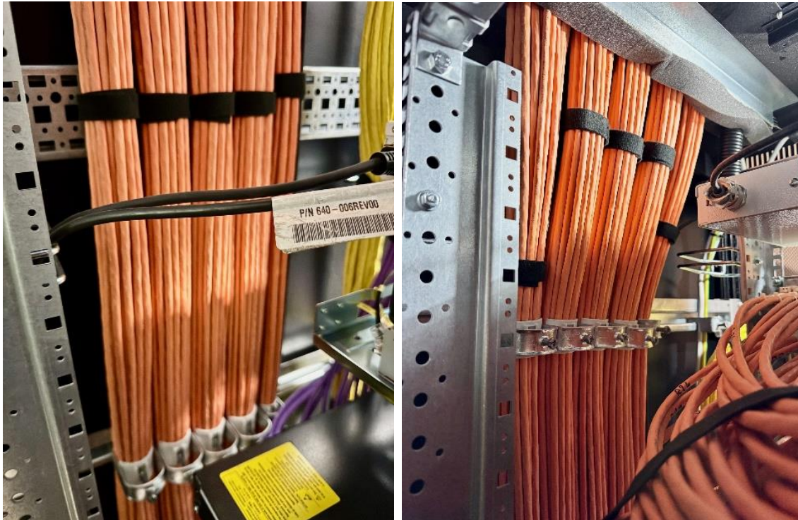
Abbildung 1: Kabelführung und Bündelung an den Seitenwänden des Schrankes
