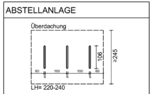
Überdachungsskizze aus dem Projektierungshandbuch der Stadt Wien
