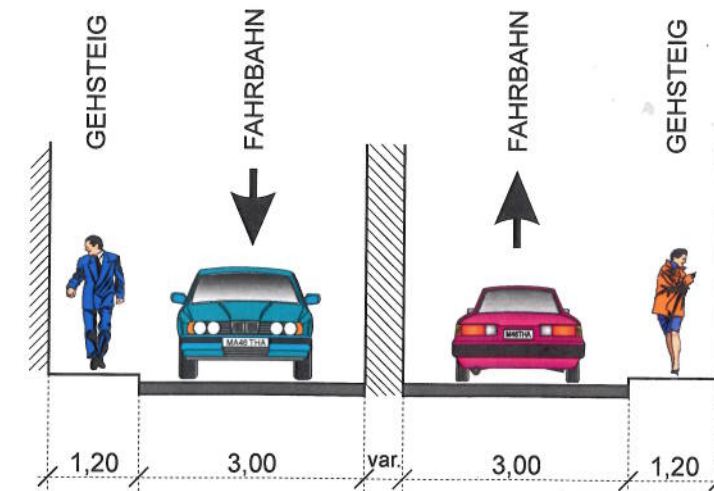
Garagen > 1.600m 2 Nutzfläche Zu- und Abfahrt mit baulicher Trennung
