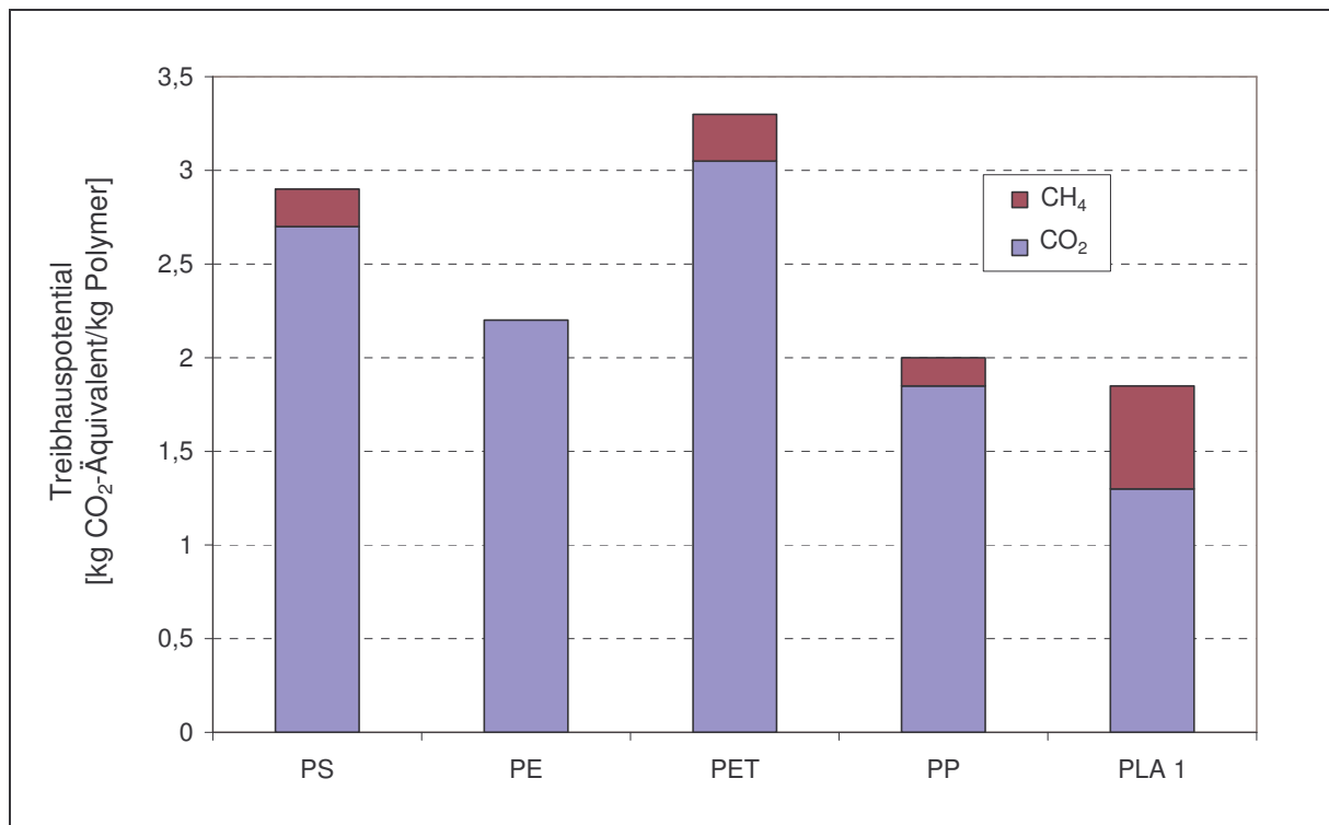
Abb. 34: Treibhauspotential bei der Herstellung von verschiedenen Kunststoffgranulaten (Quelle: Vink et al., 2003); PS...Polystyrol, PE...Polyethylen, PET...Polyethylenterephthalat, PP...Polypropylen, PLA...Polymilchsäure
