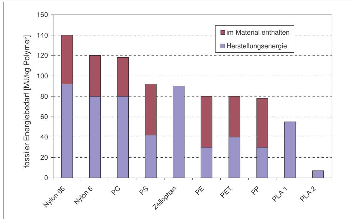
Abb. 33: Fossiler Energiebedarf zur Herstellung verschiedener Kunststoffe bis zur Granulatfertigung (Quelle: Vink et al., 2003); MJ...Megajoule, PC...Polykarbonat, PS...Polystyrol, PE...Polyethylen, PET...Polyethylenterephthalat, PP...Polypropylen, PLA...Polymilchsäure
