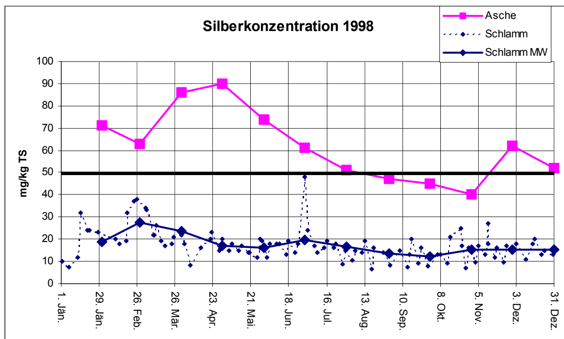
Abbildung 12-3: Ganglinien der Silberkonzentration in Wirbelschichttasche und Klärschlamm 1998; (Rohdaten: EbS)
