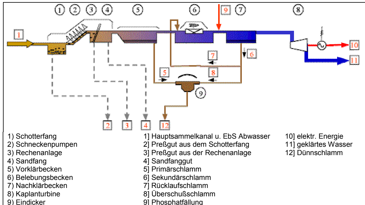
Abbildung 5-4: Hauptkläranlage Simmering
