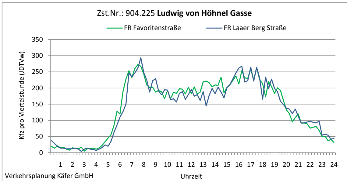
Abbildung 4-24: Tagesganglinien Ludwig von Höhnel Gasse (Zst. Nr. 904.225)
