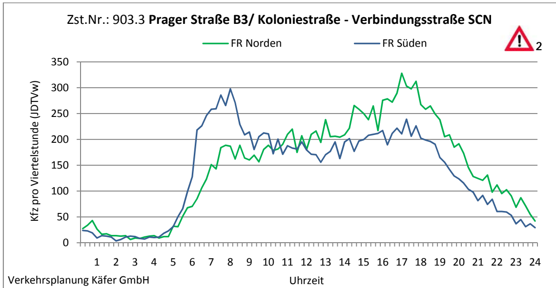
Abbildung 4-131: Tagesganglinien Prager Straße B3/ Koloniestraße - Verbindungsstraße SCN (Zst. Nr.: 903.3)
