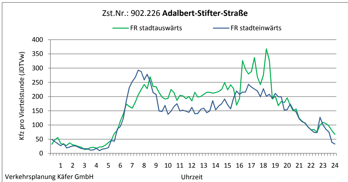
Abbildung 4-27: Tagesganglinien Adalbert-Stifter-Straße (Zst. Nr.: 902.226)
