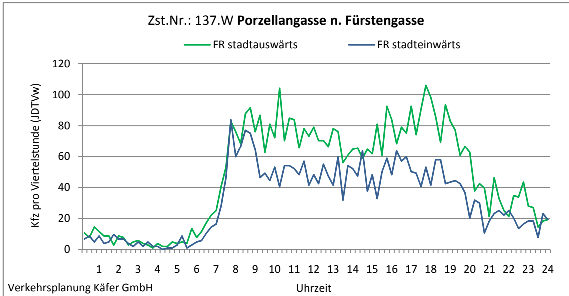
Abbildung 4-55: Tagesganglinien Porzellangasse n. Fürstengasse (Zst. Nr.: 137.W)
