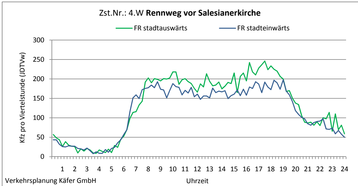
Abbildung 4-31: Tagesganglinien Rennweg vor Salesianerkirche (Zst. Nr.: 4.W)
