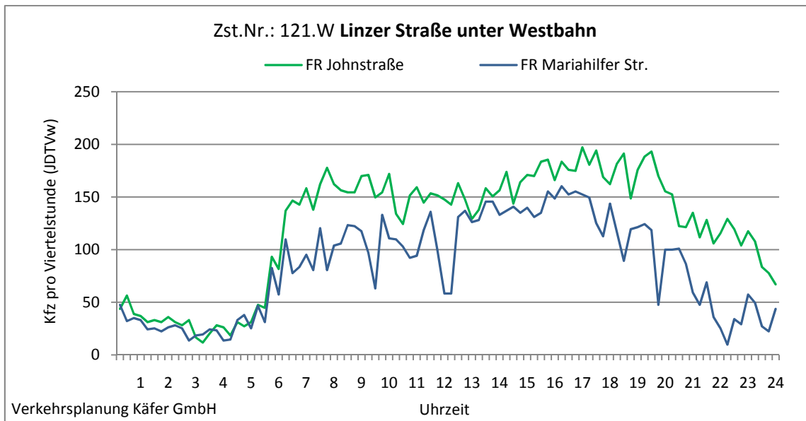
Abbildung 4-42: Tagesganglinien Linzer Straße unter Westbahn (Zst. Nr.: 121.W)
