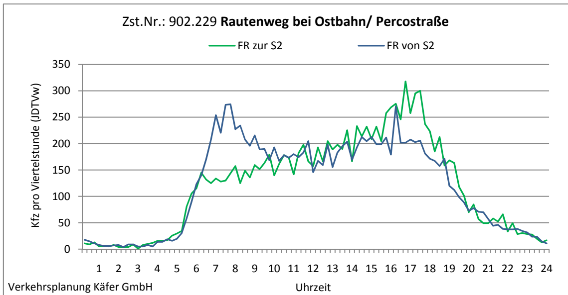
Abbildung 4-116: Tagesganglinien Rautenweg bei Ostbahn/ Percostraße (Zst. Nr.: 902.229)
