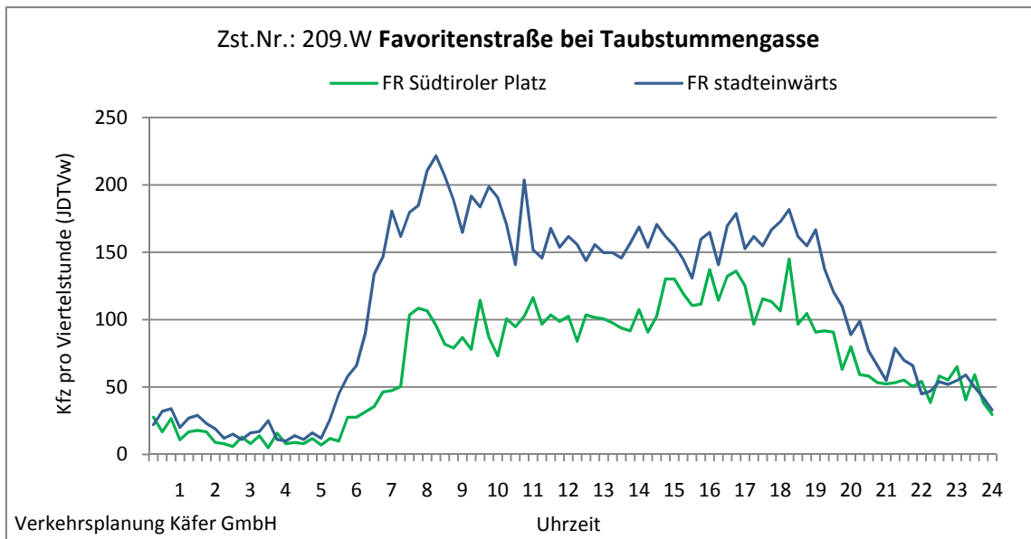
Abbildung 4-93: Tagesganglinien Favoritenstraße bei Taubstummengasse (Zst. Nr.: 209.W)
