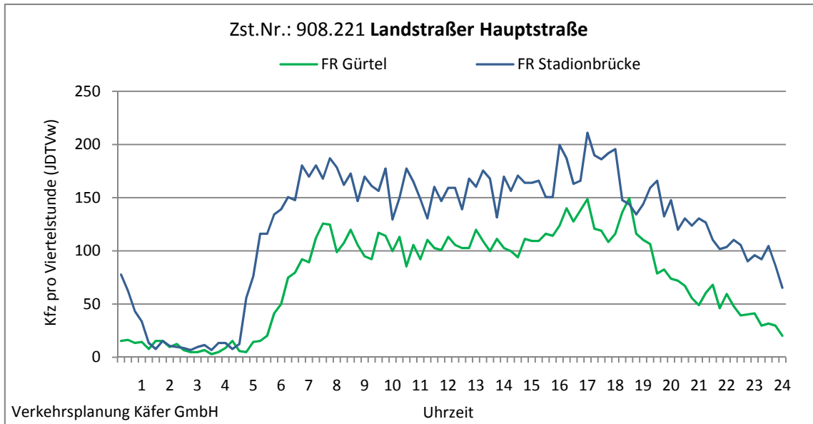
Abbildung 4-17: Tagesganglinien Landstraßer Hauptstraße (Zst. Nr.: 908.221)
