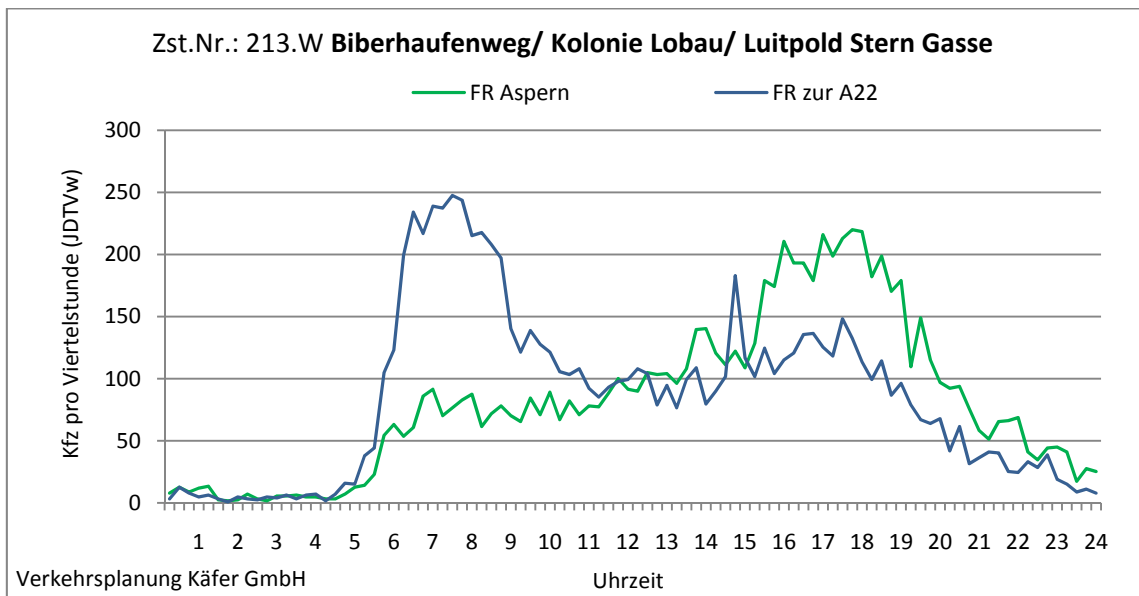
Abbildung 4-106: Tagesganglinien Biberhaufenweg/ Kolonie Lobau/ Luitpold Stern Gasse (Zst. Nr.: 213.W)
