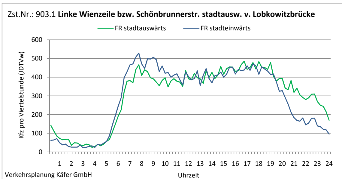
Abbildung 4-4: Tagesganglinien Linke Wienzeile bzw. Schönbrunnerstr. stadtausw. v. Lobkowitzbrücke (Zst. Nr.: 903.1)
