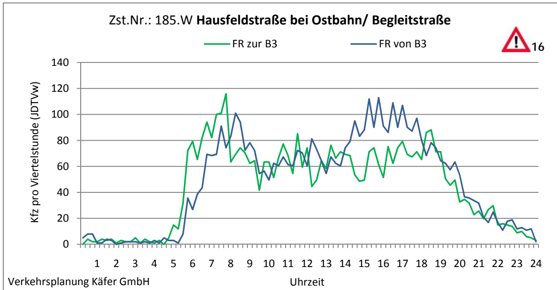
Abbildung 4-103: Tagesganglinien Hausfeldstraße bei Ostbahn/ Begleitstraße (Zst. Nr.: 185.W)
