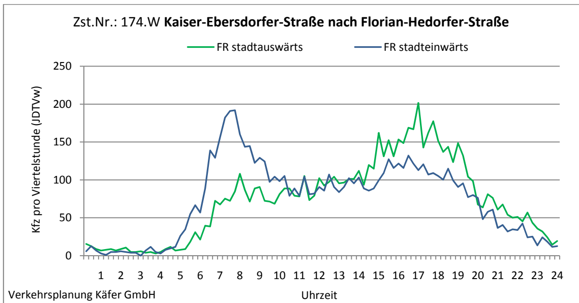
Abbildung 4-80: Tagesganglinien Kaiser-Ebersdorfer-Straße nach Florian-Hedorfer-Straße (Zst. Nr.: 174.W)
