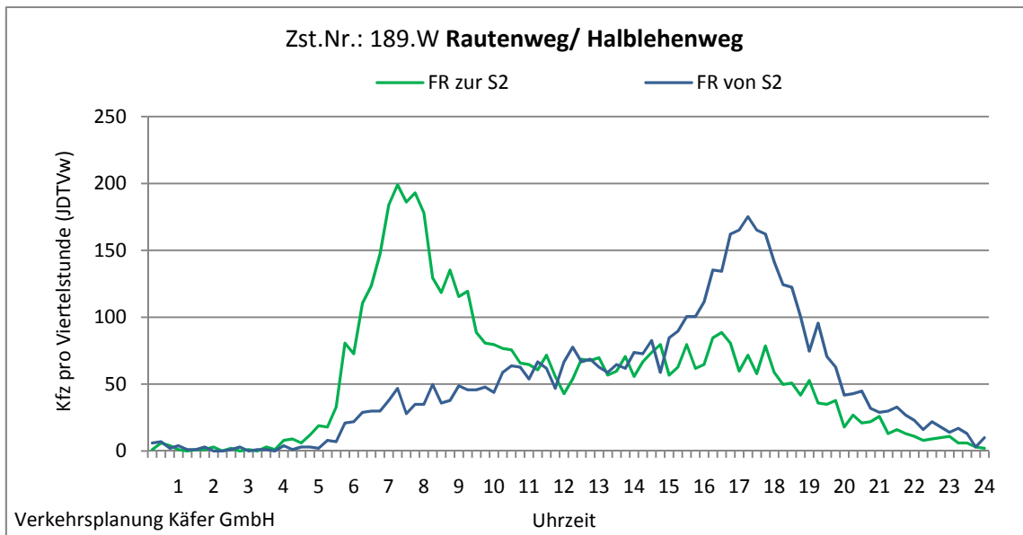
Abbildung 4-104: Tagesganglinien Rautenweg/ Halblehenweg (Zst. Nr.: 189.W)
