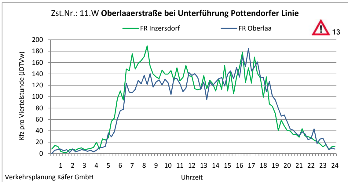
Abbildung 4-34: Tagesganglinien Oberlaaerstraße bei Unterführung Pottendorfer Linie (Zst. Nr.: 11.W)
