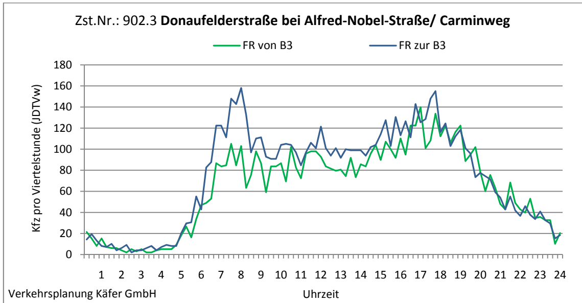
Abbildung 4-119: Tagesganglinien Donaufelderstraße bei Alfred-Nobel-Straße/ Carminweg (Zst. Nr.: 902.3)
