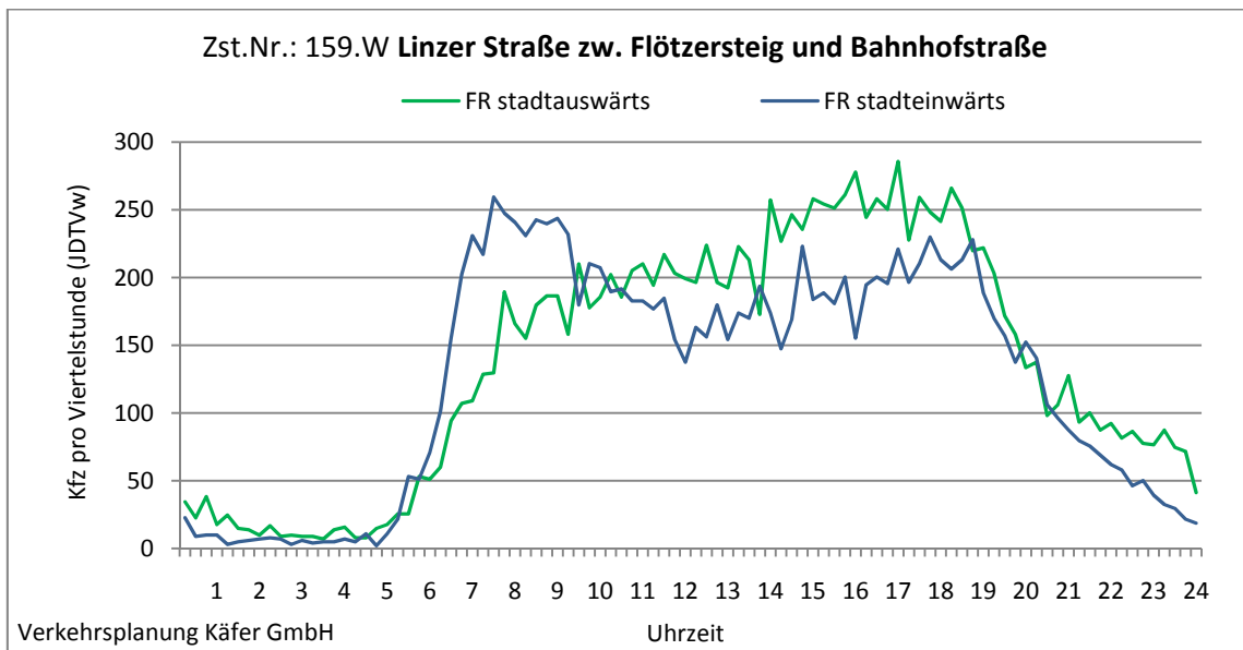
Abbildung 4-70: Tagesganglinien Linzer Straße zw. Flötzersteig und Bahnhofstraße (Zst. Nr.: 159.W)
