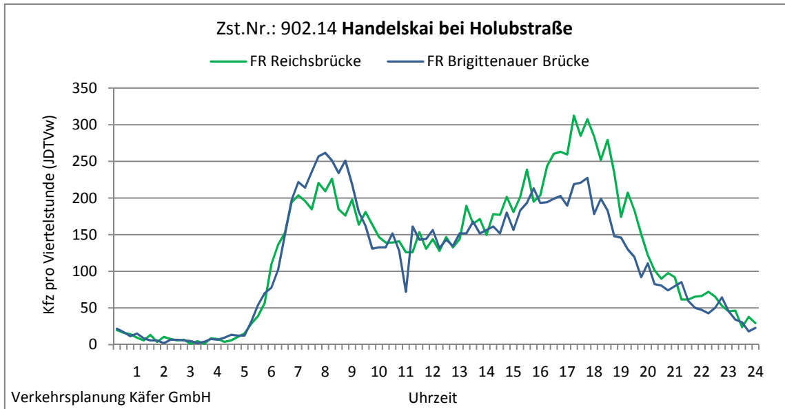
Abbildung 4-9: Tagesganglinien Handelskai bei Holubstraße (Zst. Nr.: 902.14)
