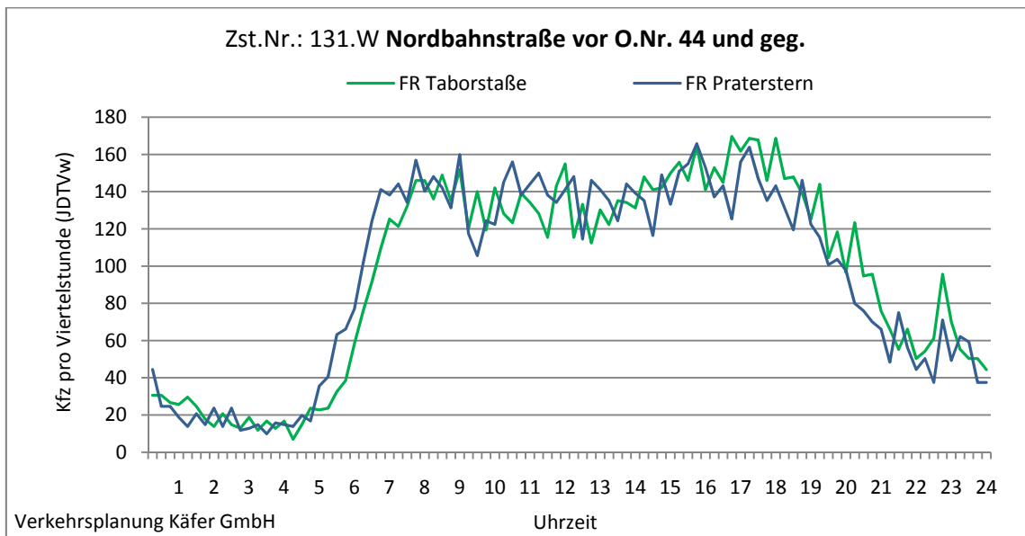
Abbildung 4-50: Tagesganglinien Nordbahnstraße vor O.Nr. 44 und geg. (Zst. Nr.: 131.W)
