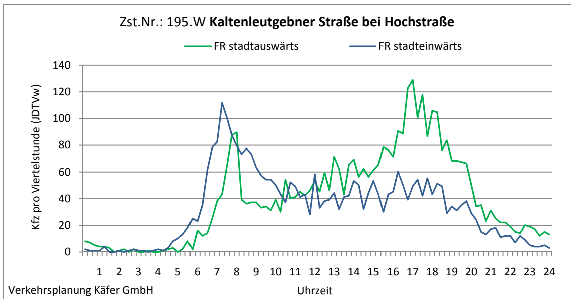
Abbildung 4-86: Tagesganglinien Kaltenleutgebner Straße bei Hochstraße (Zst. Nr.: 195.W)
