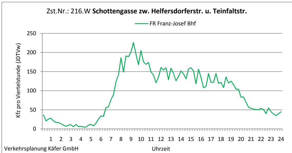
Abbildung 4-96: Tagesganglinie Schottengasse zw. Helfersdorferstr. u. Teinfaltstr. (Zst. Nr.: 216.W)
