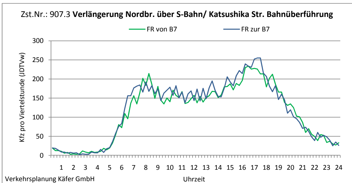
Abbildung 4-124: Tagesganglinien Verlängerung Nordbr. über S-Bahn/ Katsushika Str. Bahnüberführung (Zst.Nr.: 907.3)
