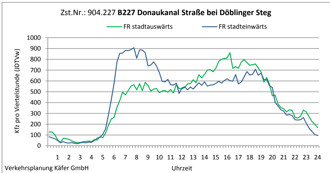
Abbildung 4-28: Tagesganglinien B227 Donaukanal Straße bei Döblinger Steg (Zst. Nr.: 904.227)
