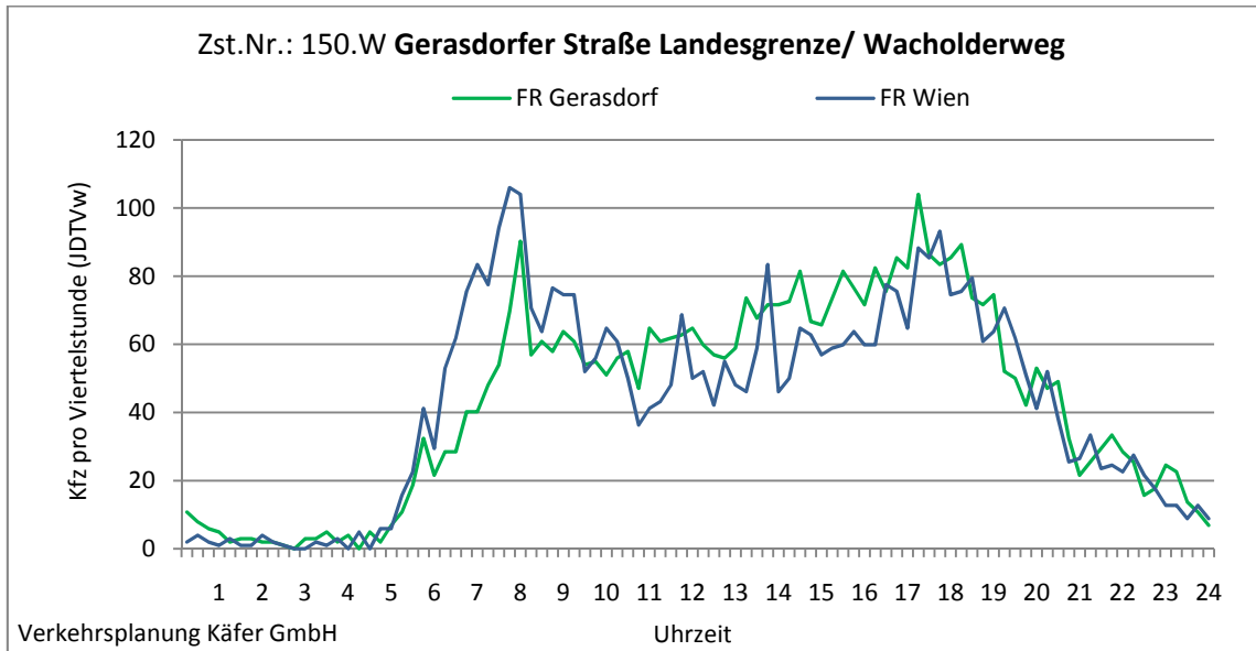
Abbildung 4-121: Tagesganglinien Gerasdorfer Straße Landesgrenze/ Wacholderweg (Zst. Nr.: 150.W)
