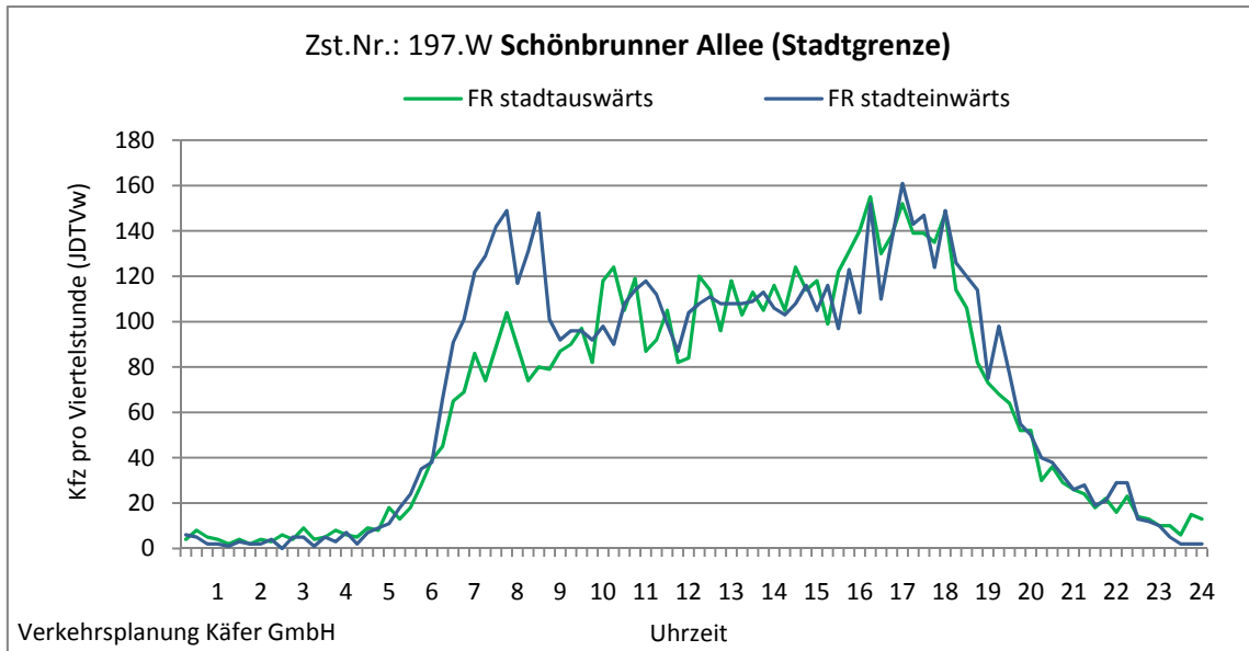
Abbildung 4-87: Tagesganglinien Schönbrunner Allee (Stadtgrenze) (Zst. Nr.: 197.W)
