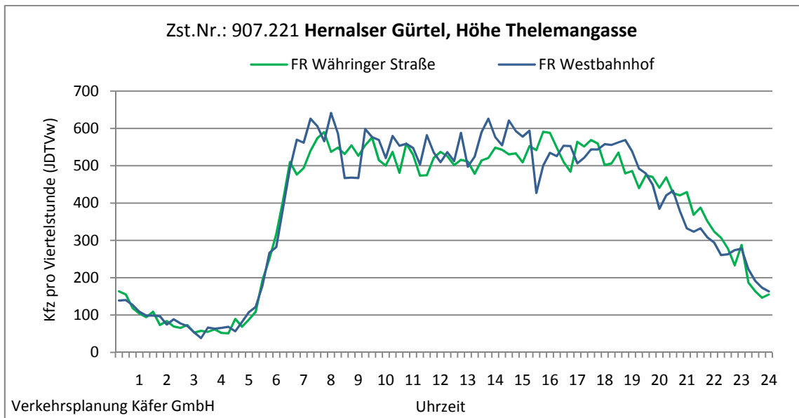
Abbildung 4-16: Tagesganglinien Hernalser Gürtel, Höhe Thelemangasse (Zst. Nr.: 907.221)
