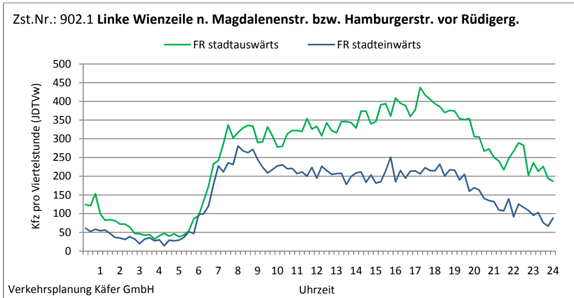
Abbildung 4-3: Tagesganglinien Linke Wienzeile n. Magdalenenstr. bzw. Hamburgerstr. vor Rüdigerg. (Zst. Nr.: 902.1)
