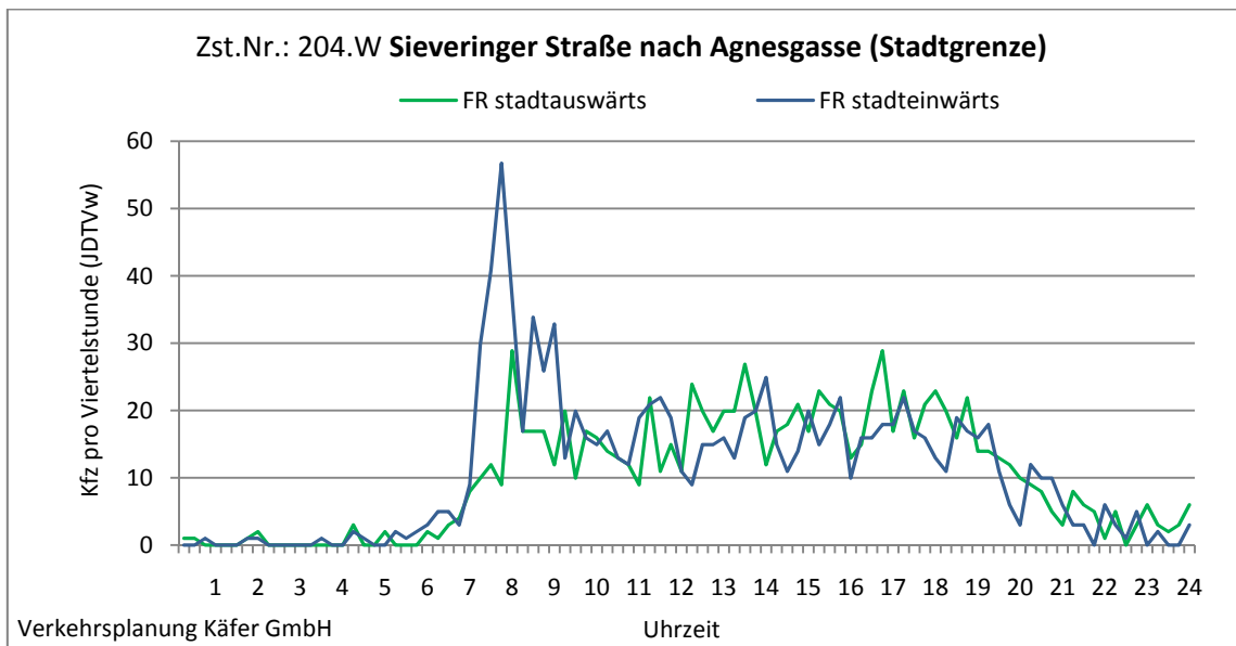
Abbildung 4-90: Tagesganglinien Sieveringer Straße nach Agnesgasse (Stadtgrenze) (Zst. Nr.: 204.W)
