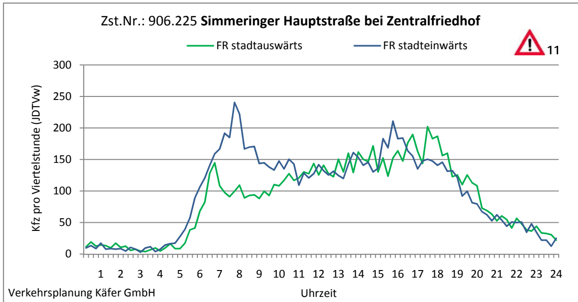
Abbildung 4-26: Tagesganglinien Simmeringer Hauptstraße bei Zentralfriedhof (Zst. Nr.: 906.225)
