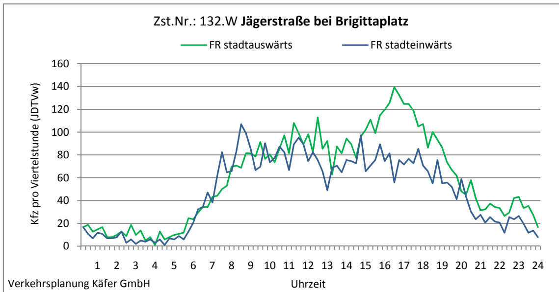
Abbildung 4-51: Tagesganglinien Jägerstraße bei Brigittaplatz (Zst. Nr.: 132.W)
