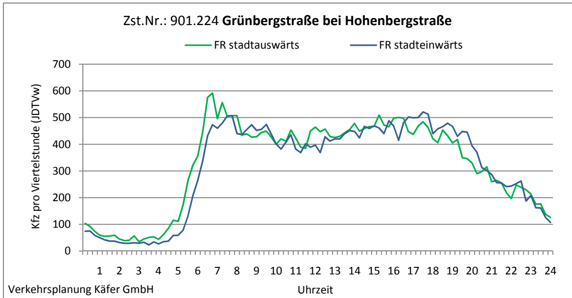
Abbildung 4-21: Tagesganglinien Grünbergstraße bei Hohenbergstraße (Zst. Nr.: 901.224)
