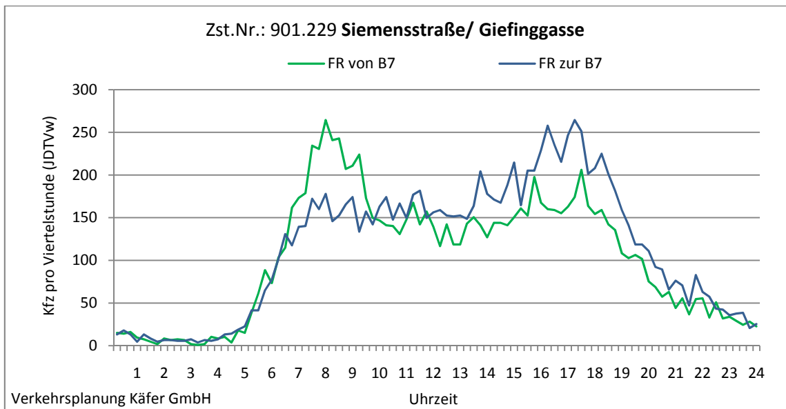
Abbildung 4-120: Tagesganglinien Siemensstraße/ Giefinggasse (Zst. Nr.: 901.229)
