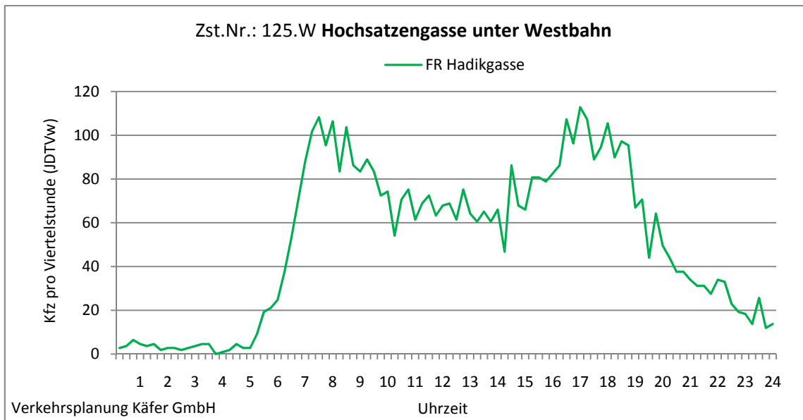
Abbildung 4-46: Tagesganglinie Hochsatzengasse unter Westbahn (Zst. Nr.: 125.W)
