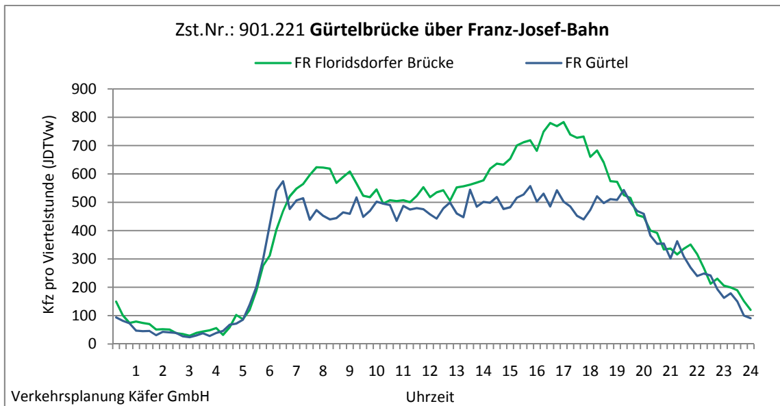
Abbildung 4-12: Tagesganglinien Gürtelbrücke über Franz-Josef-Bahn (Zst. Nr.: 901.221)
