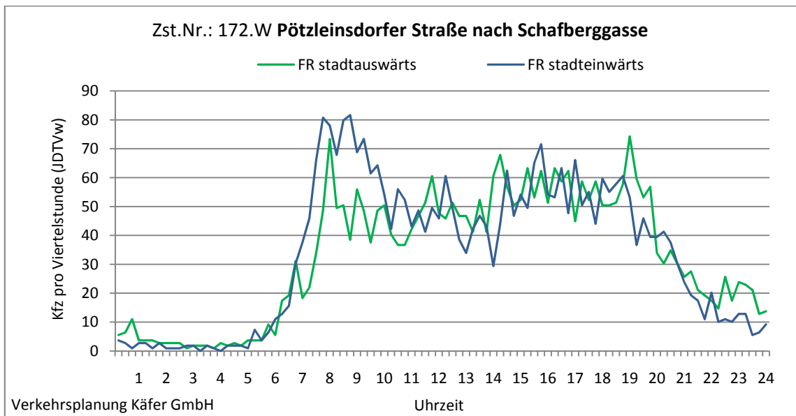
Abbildung 4-78: Tagesganglinien Pötzleinsdorfer Straße nach Schafberggasse (Zst. Nr.: 172.W)
