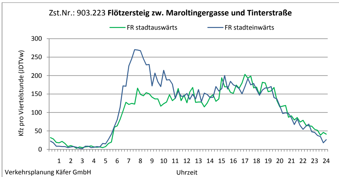
Abbildung 4-20: Tagesganglinien Flötzersteig zw. Maroltingergasse und Tinterstraße (Zst. Nr.: 903.223)
