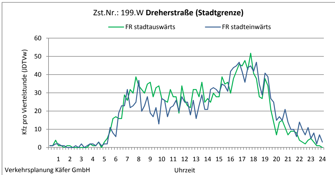
Abbildung 4-88: Tagesganglinien Dreherstraße (Stadtgrenze) (Zst. Nr.: 199.W)
