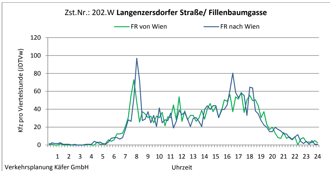
Abbildung 4-132: Tagesganglinien Langenzersdorfer Straße/ Fillenbaumgasse (Zst. Nr.: 202.W)
