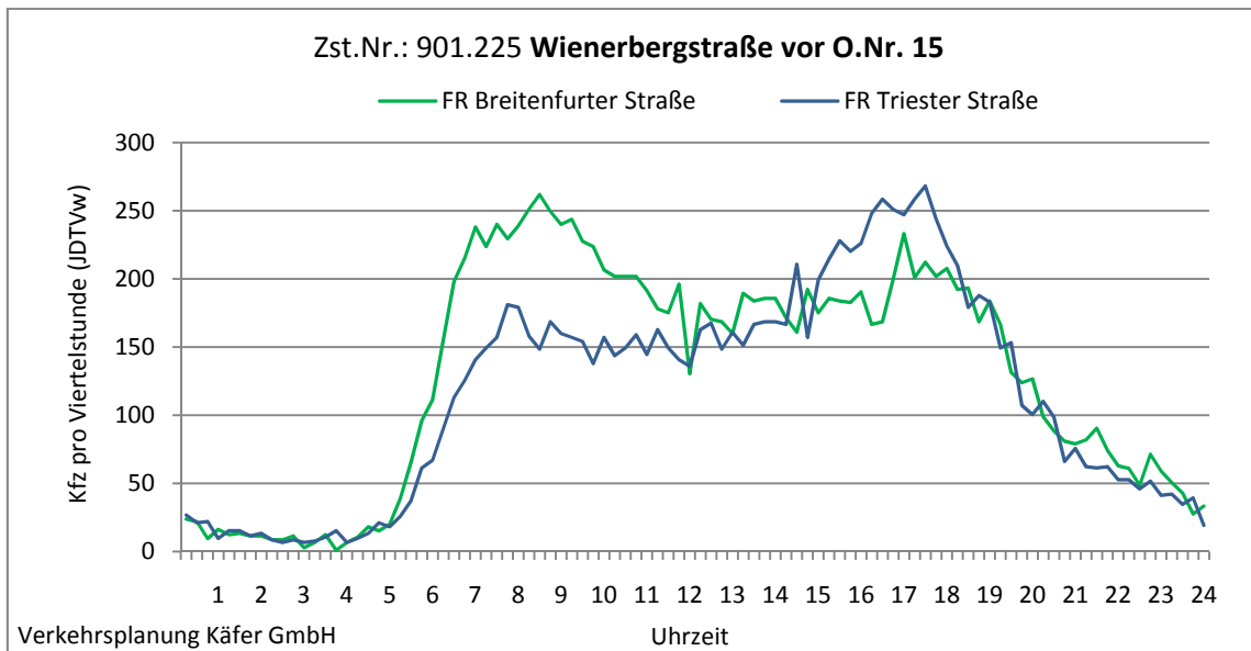
Abbildung 4-22: Tagesganglinien Wienerbergstraße vor O.Nr. 15 (Zst. Nr.: 901.225)
