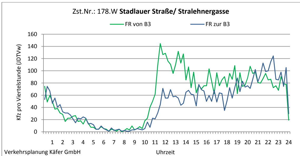
Abbildung 4-108: Tagesganglinien Stadlauer Straße/ Stralehnergasse (Zst. Nr.: 178.W)
