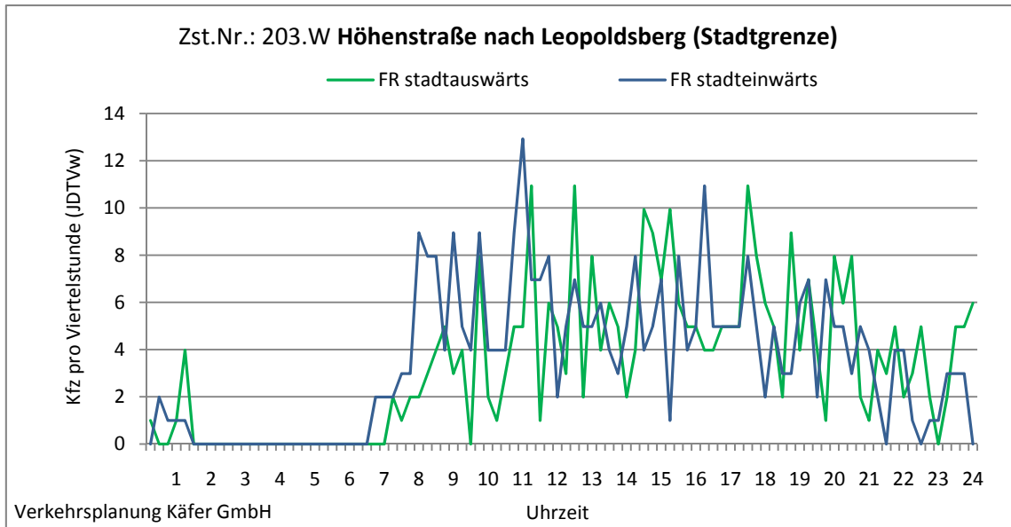
Abbildung 4-89: Tagesganglinien Höhenstraße nach Leopoldsberg (Stadtgrenze) (Zst. Nr.: 203.W)
