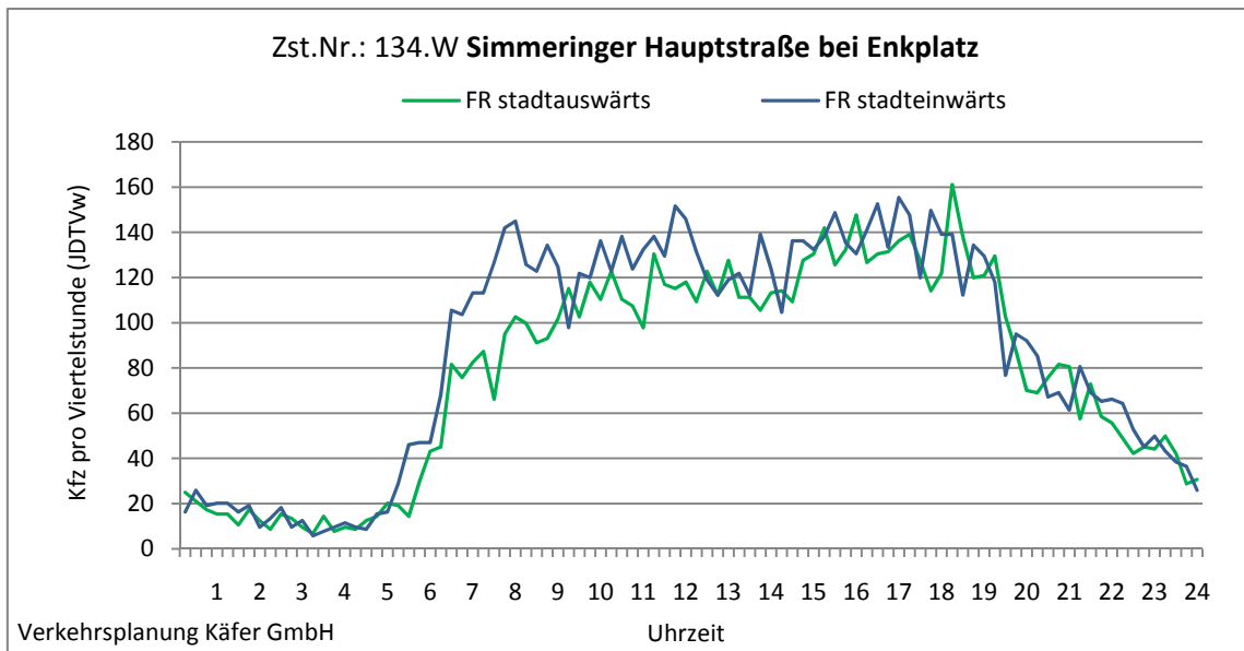
Abbildung 4-53: Tagesganglinien Simmeringer Hauptstraße bei Enkplatz (Zst. Nr.: 134.W)
