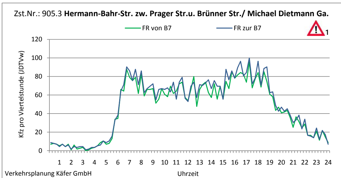
Abbildung 4-126: Tagesganglinien Hermann-Bahr-Str. zw. Prager Str. u. Brünner Str./ Michael Dietmann Gasse (Zst. Nr.: 905.3)
