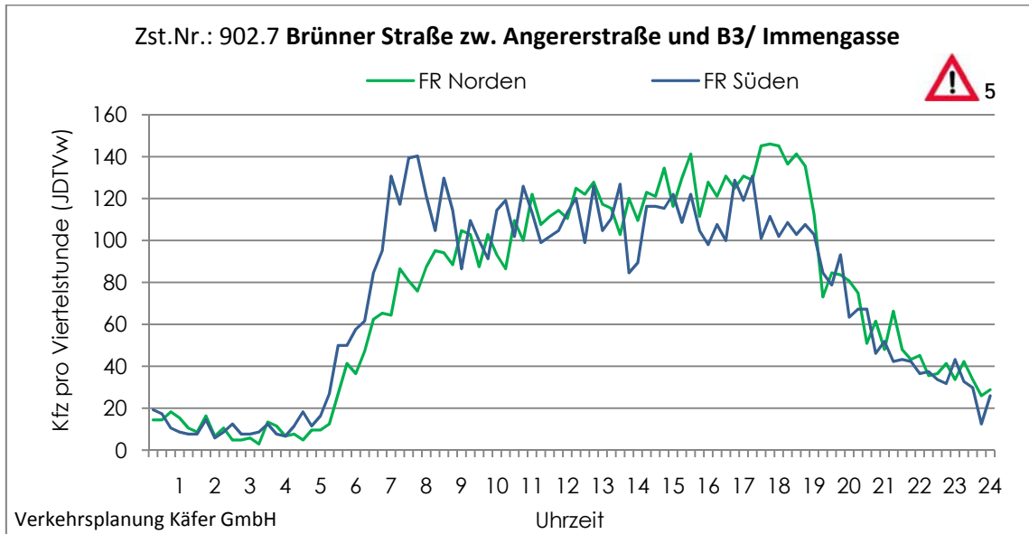
Abbildung 4-127: Tagesganglinien Brünner Straße zw. Angererstraße und B3/ Immengasse (Zst. Nr.: 902.7)
