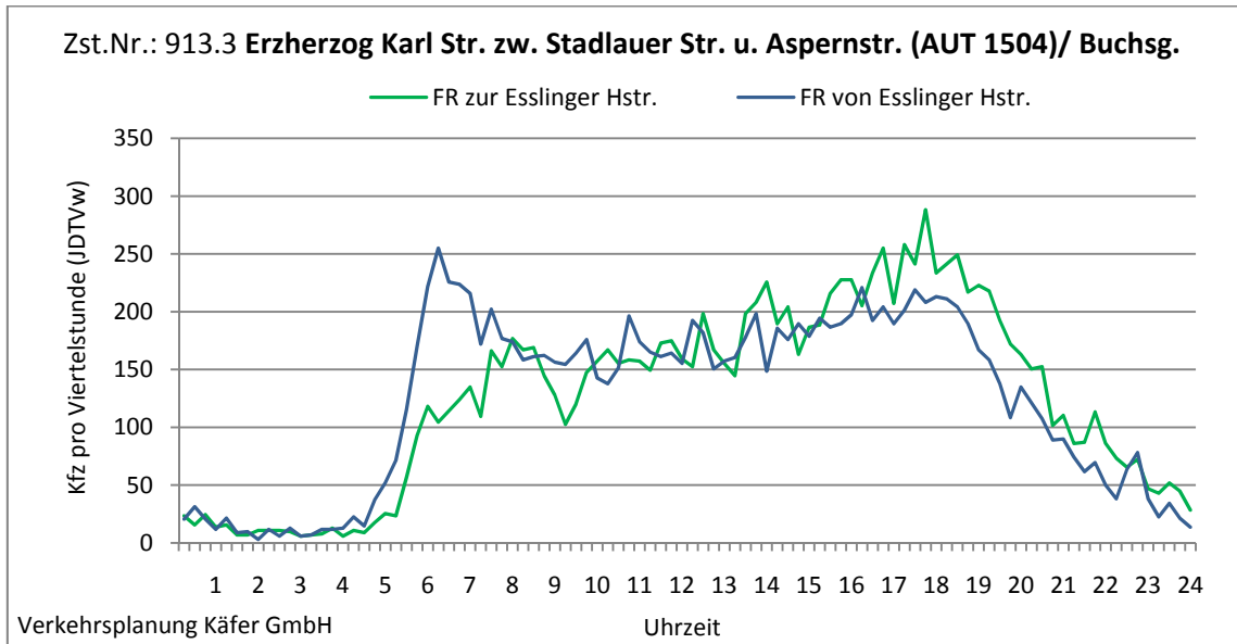
Abbildung 4-101: Erzherzog-Karl-Straße zw. Stadlauer Str. u. Aspernstr. (Aut 1504)/ Buchsg. (Zst. Nr.: 913.3)
