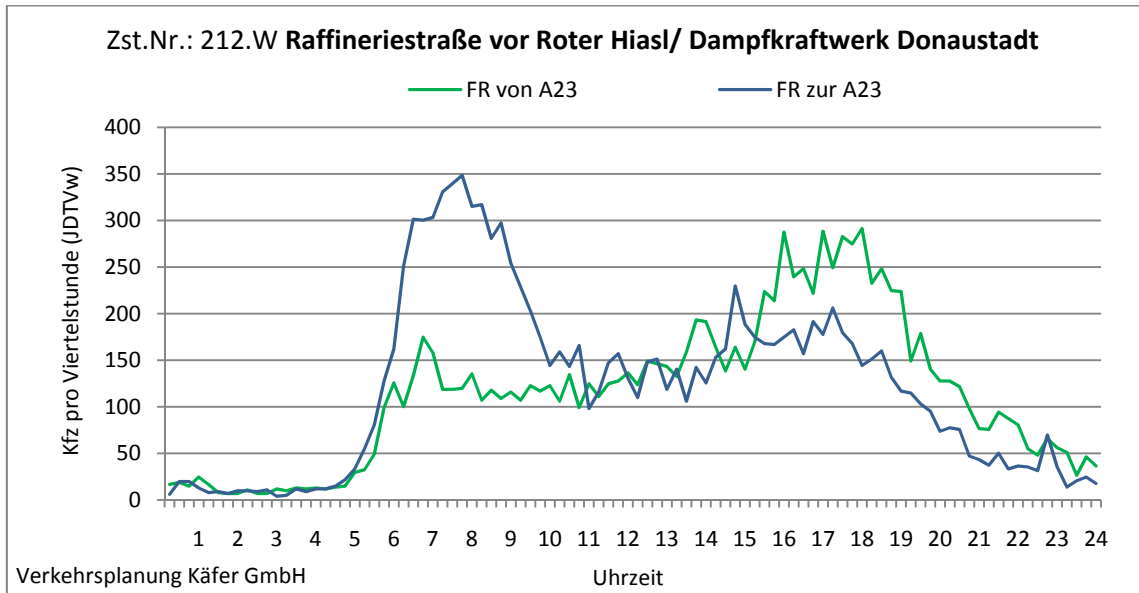
Abbildung 4-107: Tagesganglinien Raffineriestraße vor Roter Hiasl/ Dampfkraftwerk Donaustadt (Zst. Nr.: 212.W)
