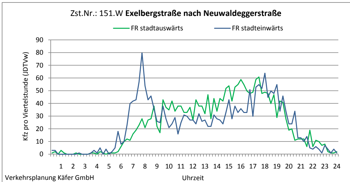
Abbildung 4-64: Tagesganglinien Exelbergstraße nach Neuwaldeggerstraße (Zst. Nr.: 151.W)
