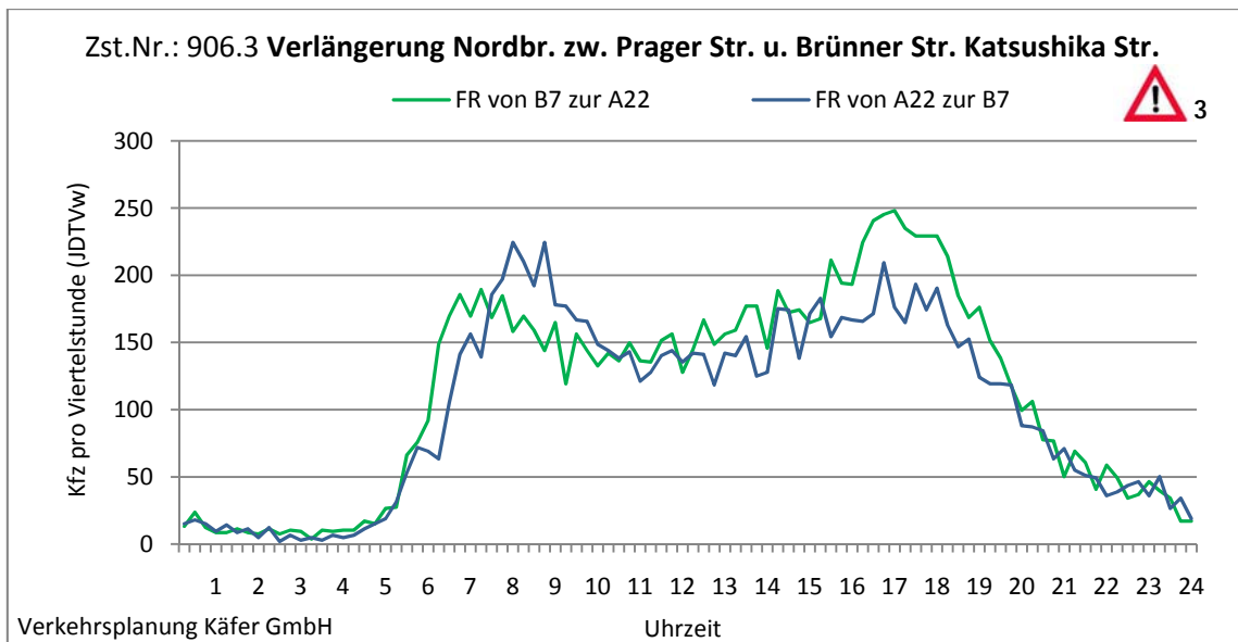
Abbildung 4-128: Tagesganglinien Verlängerung Nordbr. zw. Prager Str. u. Brünner Str. Katsushika Str. (Zst. Nr.: 906.3)
