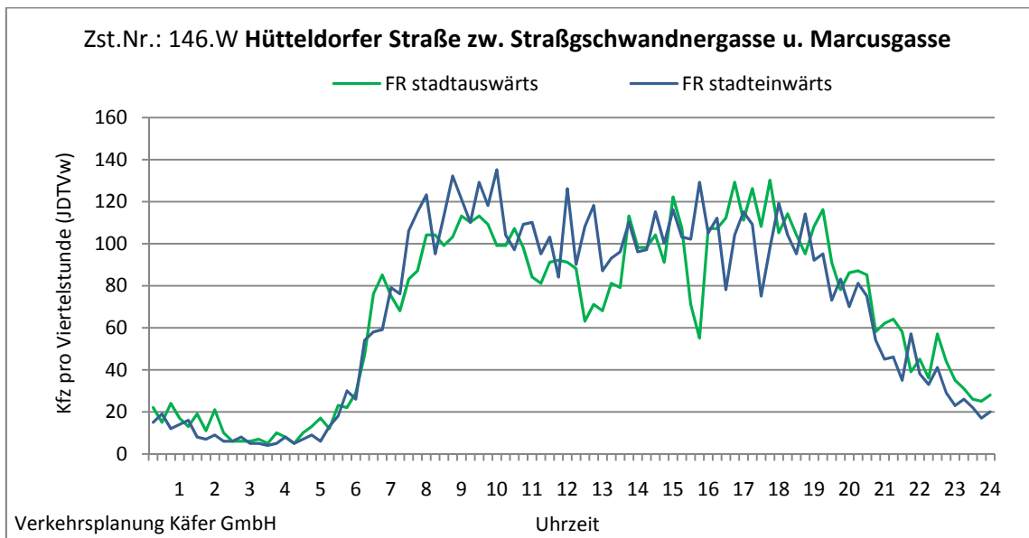
Abbildung 4-62: Tagesganglinien Hütteldorfer Straße zw. Straßschwandnergasse u. Marcusgasse (Zst. Nr.: 146.W)
