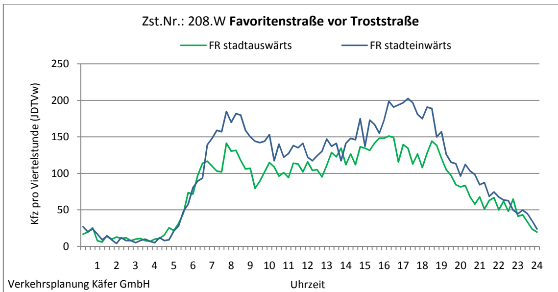
Abbildung 4-92: Tagesganglinien Favoritenstraße vor Troststraße (Zst. Nr.: 208.W)
