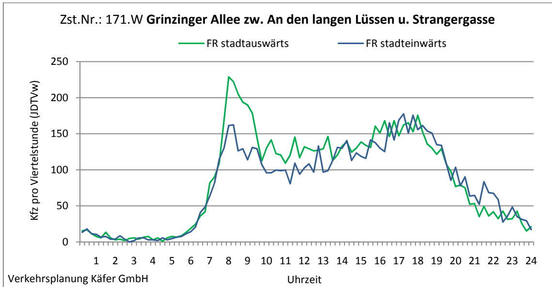
Abbildung 4-77: Tagesganglinien Grinzinger Allee zw. An den langen Lüssen u. Strangergasse (Zst. Nr.: 171.W)
