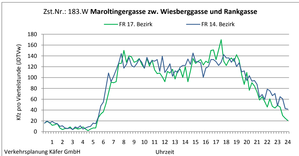
Abbildung 4-84: Tagesganglinien Maroltingergasse zw. Wiesberggasse und Rankgasse (Zst. Nr.: 183.W)
