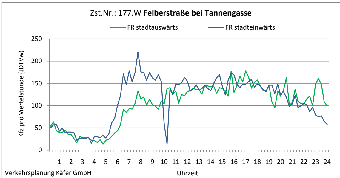
Abbildung 4-81: Tagesganglinien Felberstraße bei Tannengasse (Zst. Nr.: 177.W)
