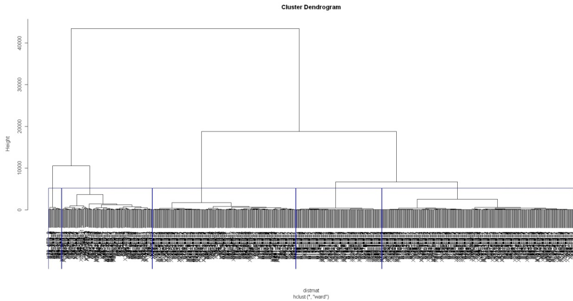
Abbildung 3-3: Clusteranalyse – Dendrogramm Fzg-Gruppe bis 12m
