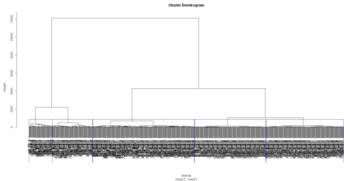
Abbildung 3-4: Clusteranalyse – Dendrogramm Fzg-Gruppe > 12m
