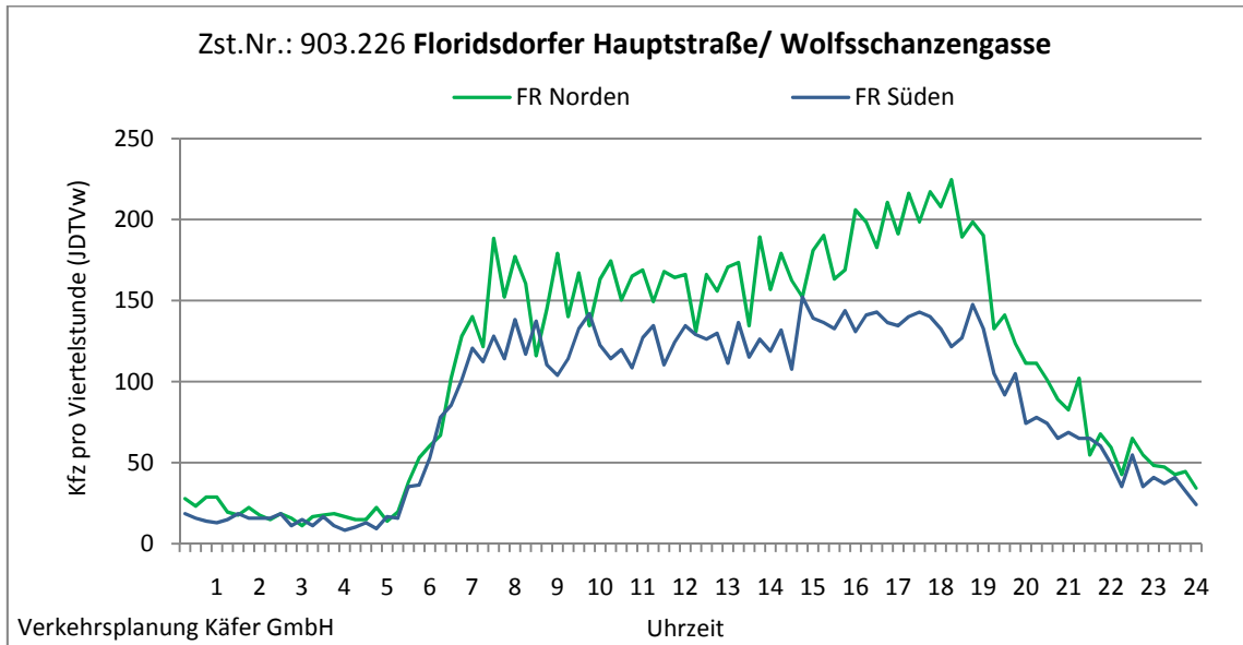
Abbildung 4-125: Tagesganglinien Floridsdorfer Hauptstraße/ Wolfsschanzengasse (Zst. Nr.: 903.226)
