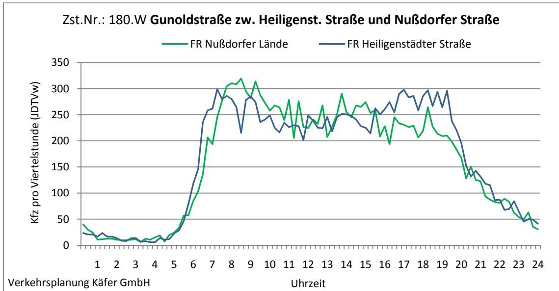
Abbildung 4-83: Tagesganglinien Gunoldstraße zw. Heilingst. Straße und Nußdorfer Straße (Zst. Nr.: 180.W)
