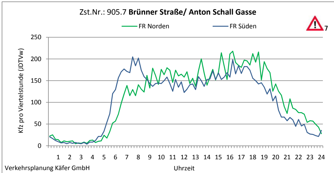
Abbildung 4-133: Tagesganglinien Brünner Straße/ Anton Schall Gasse (Zst. Nr.: 905.7)
