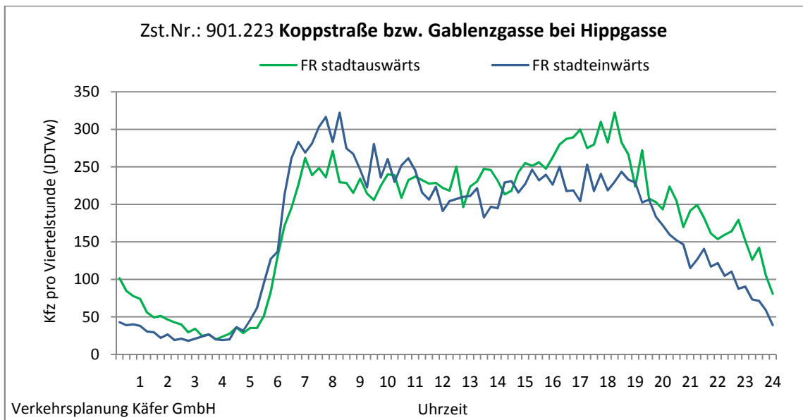
Abbildung 4-18: Tagesganglinien Koppstraße bzw. Gablenzgasse bei Hippgasse (Zst. Nr.: 901.223)
