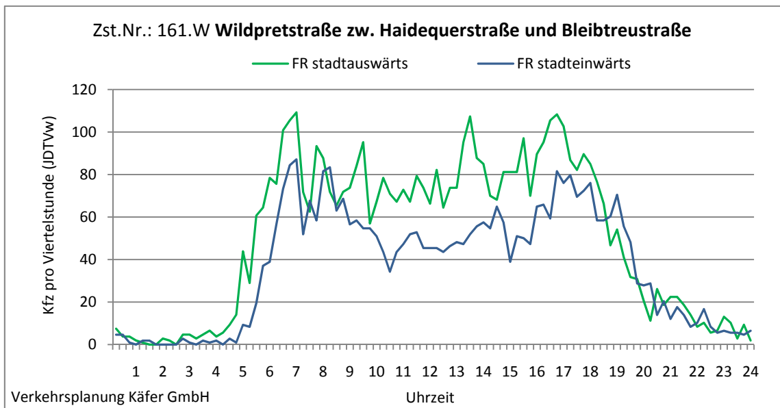
Abbildung 4-72: Tagesganglinien Wildpretstraße zw. Haidequerstraße und Bleibtreststraße (Zst. Nr.: 161.W)
