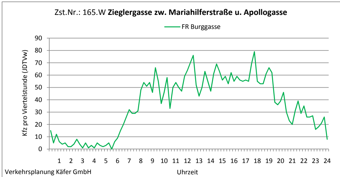
Abbildung 4-75: Tagesganglinie Zieglergasse zw. Mariahilferstraße u. Apollogasse (Zst. Nr.: 165.W)
