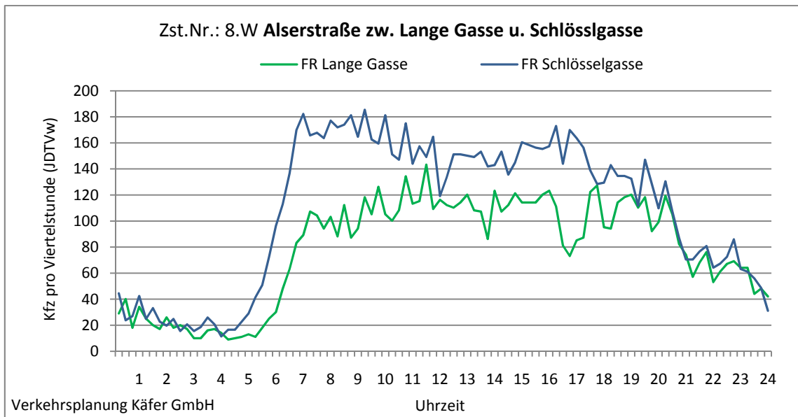
Abbildung 4-32: Tagesganglinien Alserstraße zw. Lange Gasse u. Schöllgasse (Zst. Nr. 8.W)
