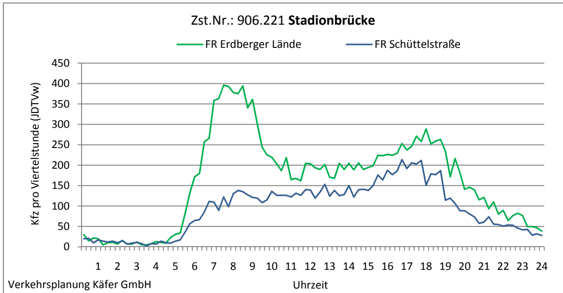
Abbildung 4-15: Tagesganglinien Stadionbrücke (Zst. Nr.: 906.221)
