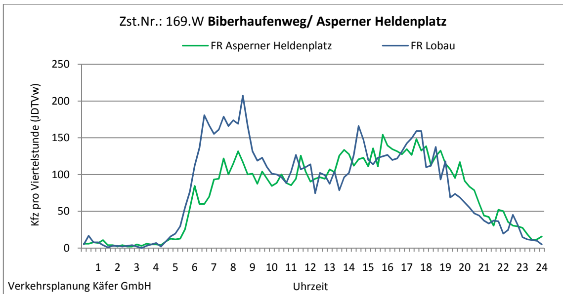
Abbildung 4-100: Tagesganglinien Biberhaufenweg/ Asperner Heldenplatz (Zst. Nr.: 169.W)
