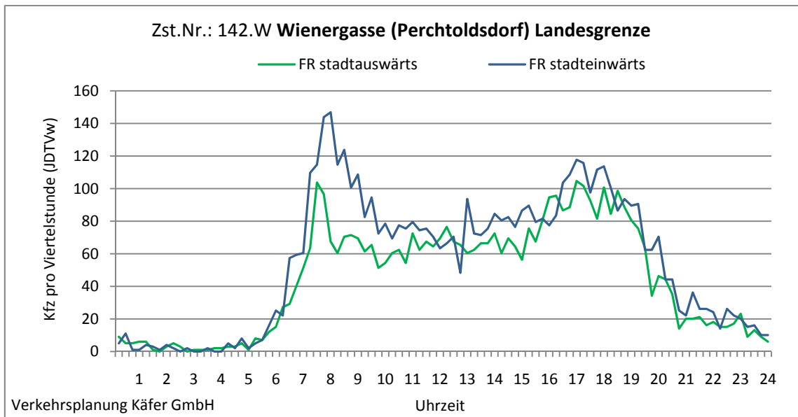
Abbildung 4-58: Tagesganglinien Wienergasse (Perchtoldsdorf) Landesgrenze (Zst. Nr.: 142.W)
