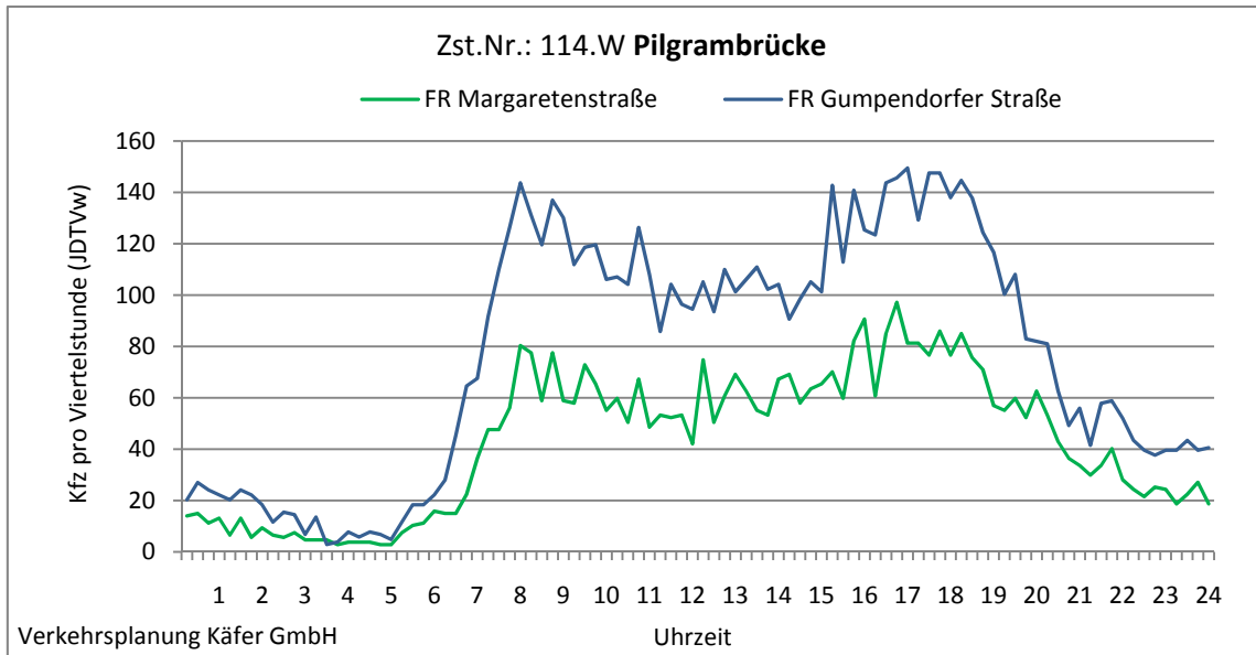
Abbildung 4-39: Tagesganglinien Pilgrambrücke (Zst. Nr.: 114.W)
