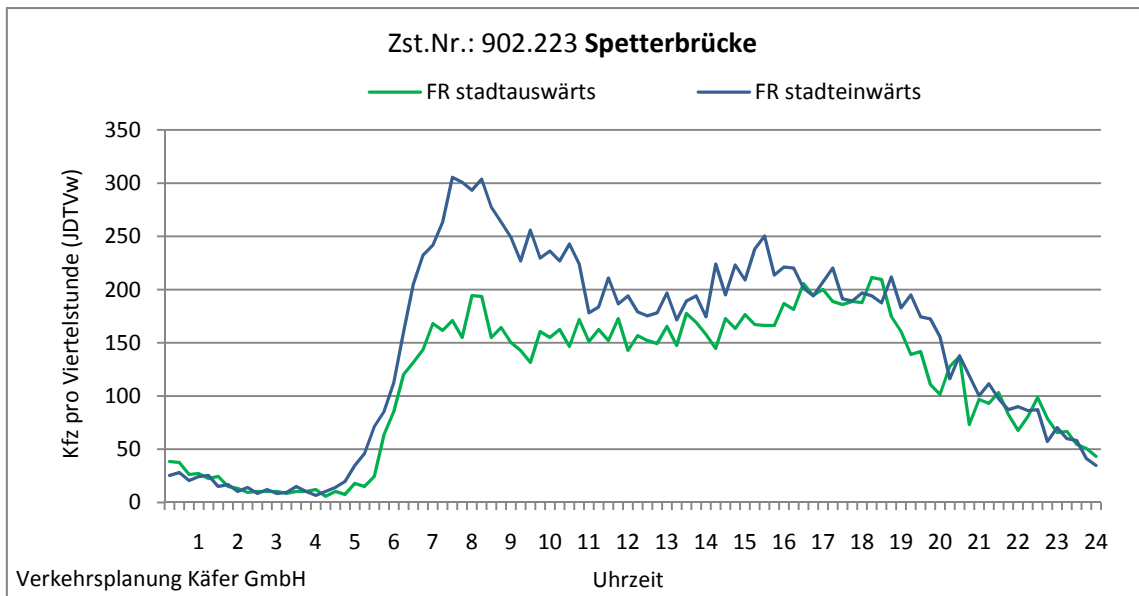
Abbildung 4-19: Tagesganglinien Spetterbrücke (Zst. Nr.: 902.223)
