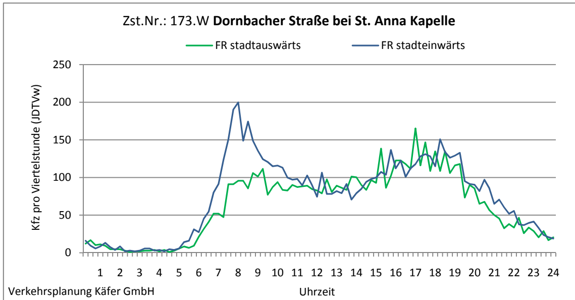
Abbildung 4-79: Tagesganglinien Dornbacher Straße bei St. Anna Kapelle (Zst. Nr.: 173.W)
