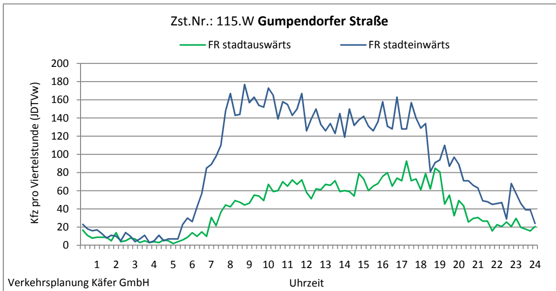
Abbildung 4-40: Tagesganglinien Gumpendorfer Straße (Zst. Nr.: 115.W)
