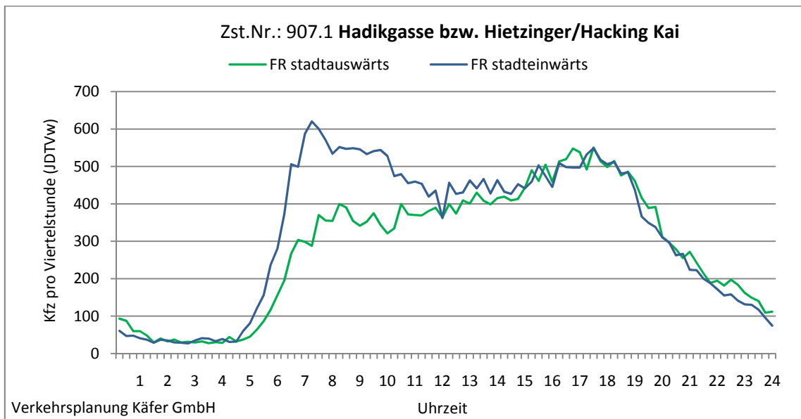
Abbildung 4-6: Tagesganglinien Hadikgasse bzw. Hietzinger/Hacking Kai (Zst. Nr.: 907.1)
