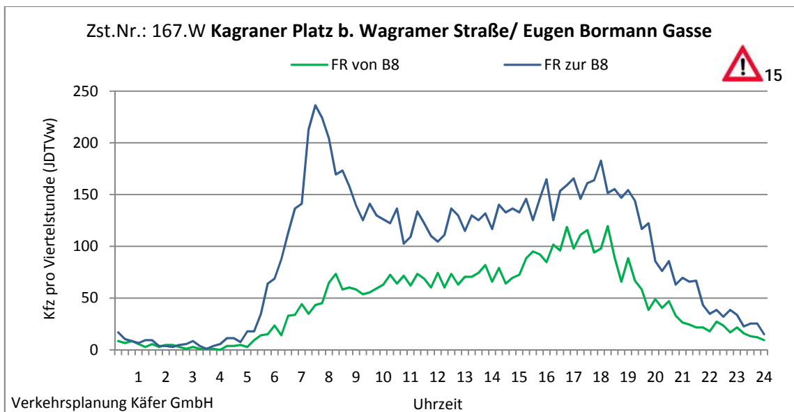
Abbildung 4-110: Tagesganglinien Kagraner Platz b. Wagramer Straße/ Eugen Bormann Gasse (Zst. Nr.: 167.W)
