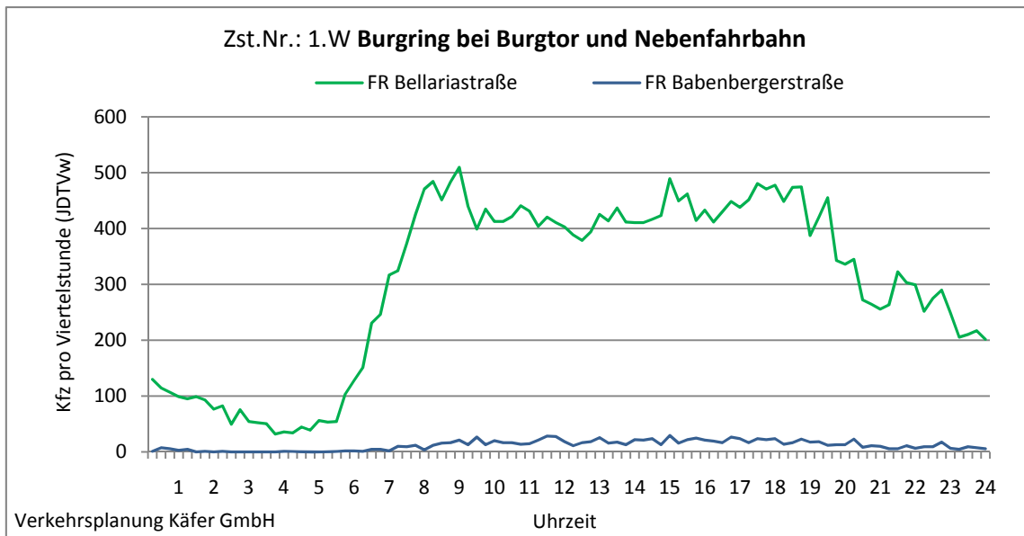
Abbildung 4-29: Tagesganglinien Burgring bei Burgtor und Nebenfahrbahn (Zst. Nr.: 1.W)
