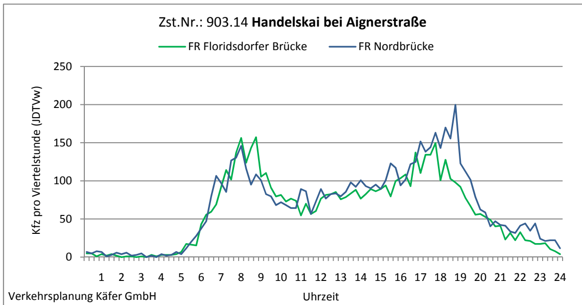
Abbildung 4-10: Tagesganglinien Handelskai bei Aignerstraße (Zst. Nr.: 903.14)
