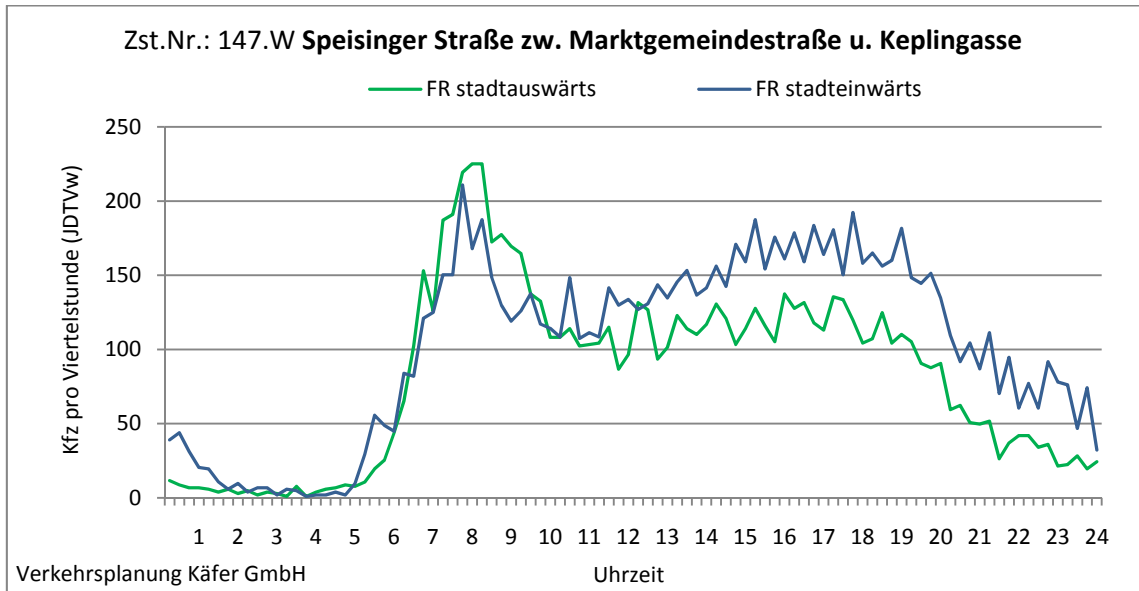
Abbildung 4-63: Tagesganglinien Speisinger Straße zw. Martgemeindestraße u. Keplingasse (Zst. Nr.: 147.W)
