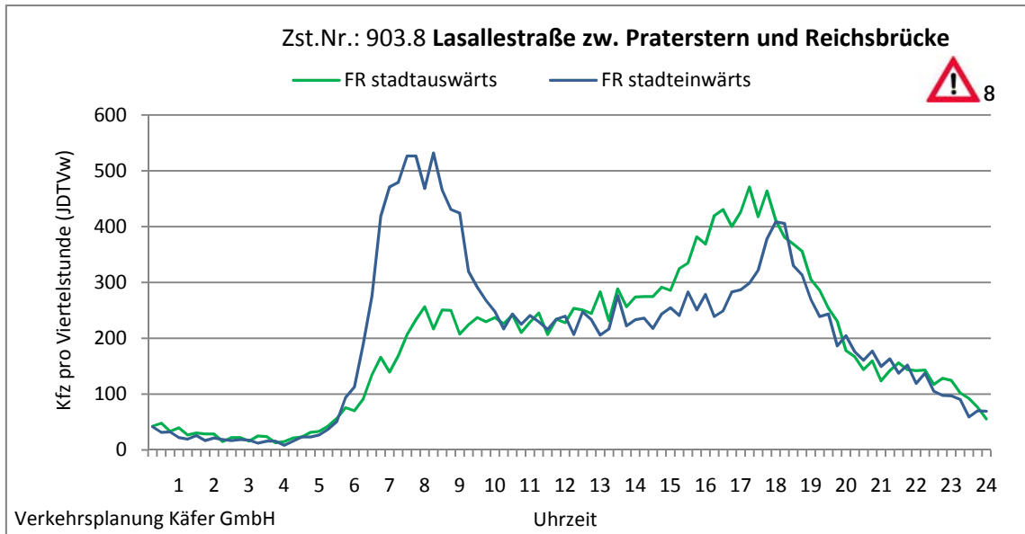
Abbildung 4-7: Tagesganglinien Lasallestraße zw. Praterstern und Reichsbrücke (Zst. Nr.: 903.8)
