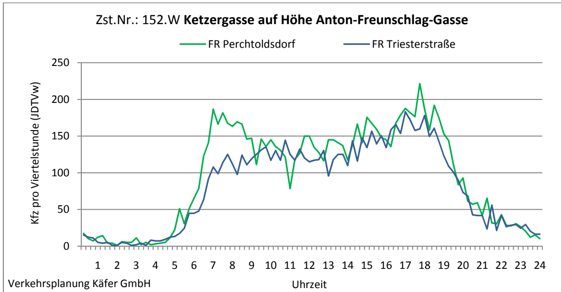
Abbildung 4-65: Tagesganglinien Ketzergasse auf Höhe Anton-Freunschlag-Gasse (Zst. Nr.: 152.W)
