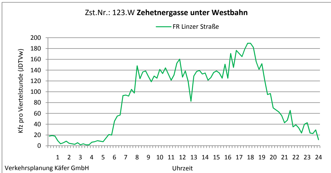
Abbildung 4-44: Tagesganglinie Zehetnergasse unter Westbahn (Zst. Nr.: 123.W)
