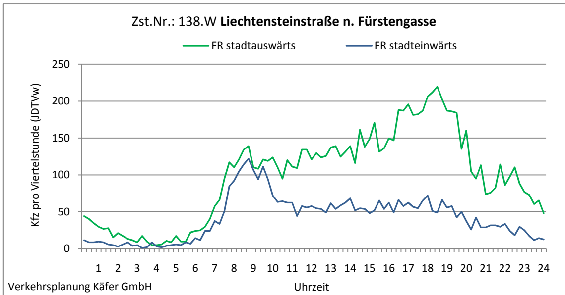
Abbildung 4-56: Tagesganglinien Liechtensteinstraße n. Fürstengasse (Zst. Nr.: 138.W)
