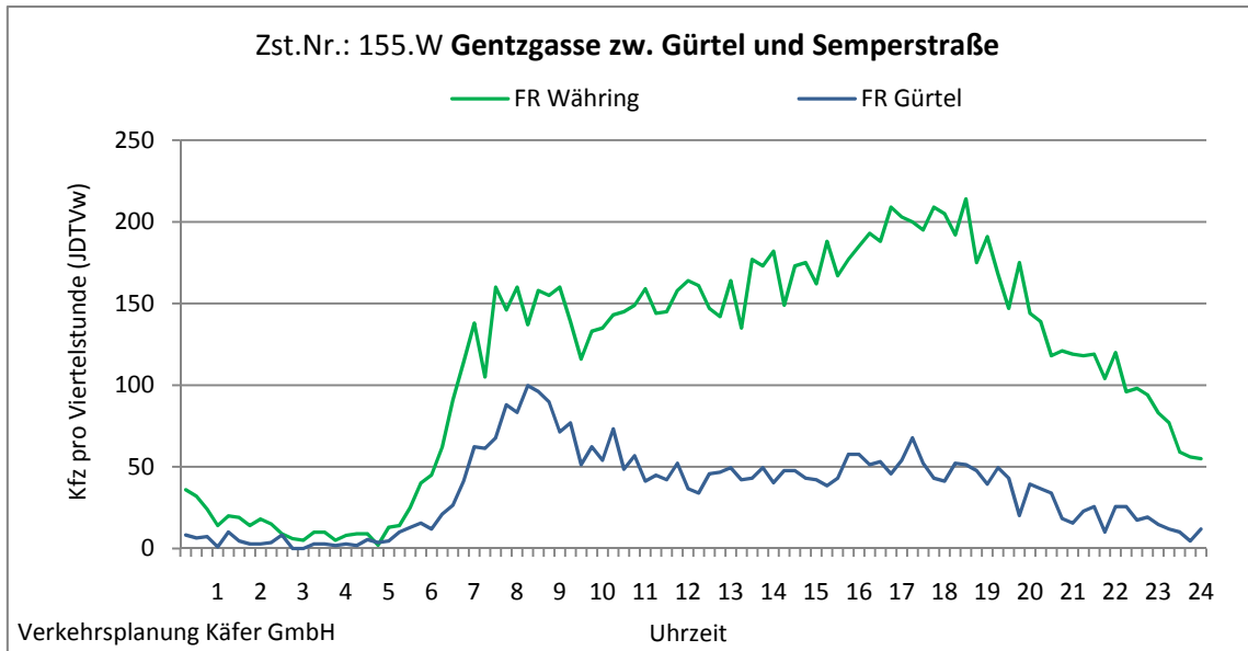
Abbildung 4-67: Tagesganglinien Gentzgasse zw. Gürtel und Semperstraße (Zst. Nr.: 155.W)
