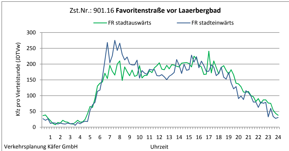
Abbildung 4-11: Tagesganglinien Favoritenstraße vor Laaerbergbad (Zst. Nr.: 901.16)
