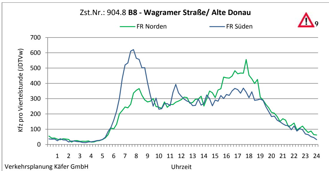
Abbildung 4-112: Tagesganglinien B8 Wagramer Straße/ Alte Donau (Zst. Nr.: 904.8)
