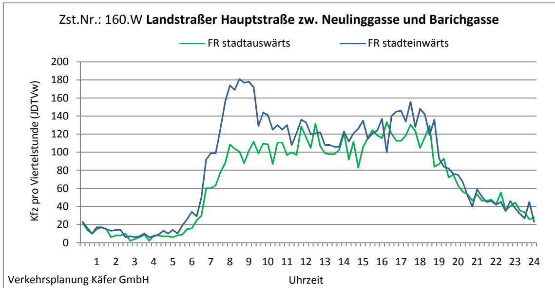
Abbildung 4-71: Tagesganglinien Landstraßer Hauptstraße zw. Neulinggasse und Barichgasse (Zst. Nr.: 160.W)
