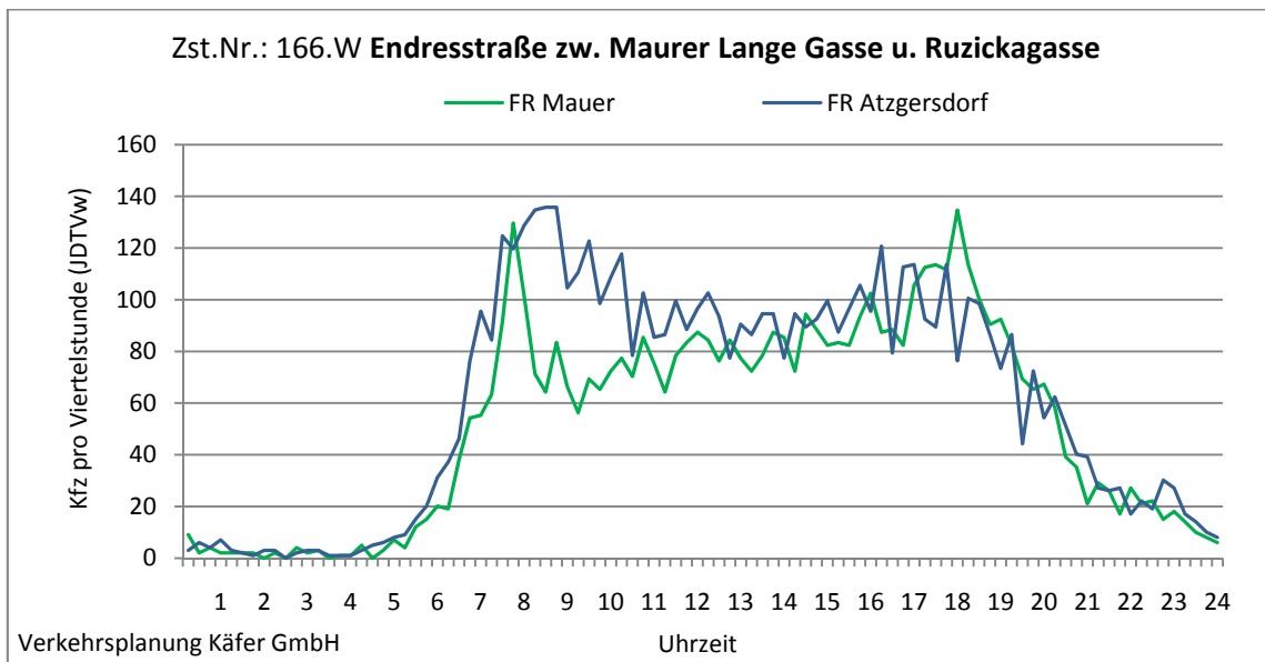
Abbildung 4-76: Tagesganglinien Endresstraße zw. Maurer Lange Gasse u. Ruzickagasse (Zst. Nr. 166.W)
