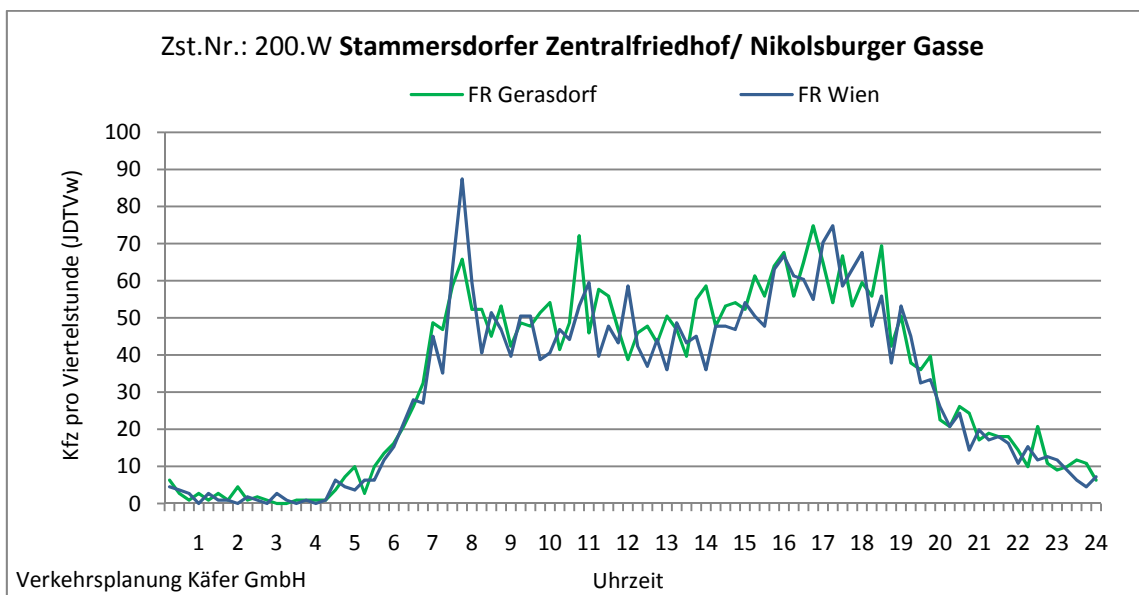
Abbildung 4-122: Tagesganglinien Stammersdorfer Zentralfriedhof/ Nikolsburger Gasse (Zst. Nr.: 200.W)
