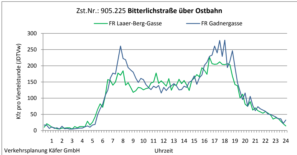
Abbildung 4-25: Tagesganglinien Bitterlichstraße über Ostbahn (Zst. Nr.: 905.225)
