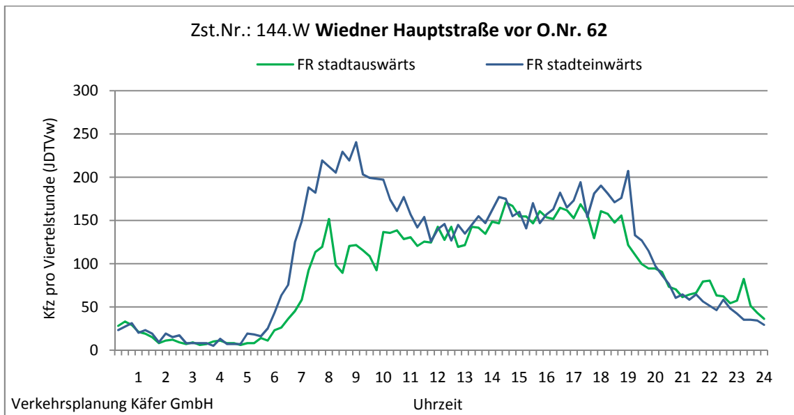
Abbildung 4-60: Tagesganglinien Wiedner Hauptstraße vor O.Nr. 62 (Zst. Nr.: 144.W)
