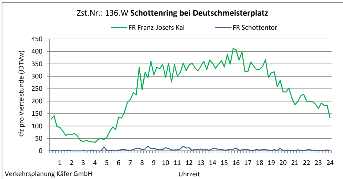
Abbildung 4-54: Tagesganglinien Schottenring bei Deutschmeisterplatz (Zst. Nr.: 136.W)
