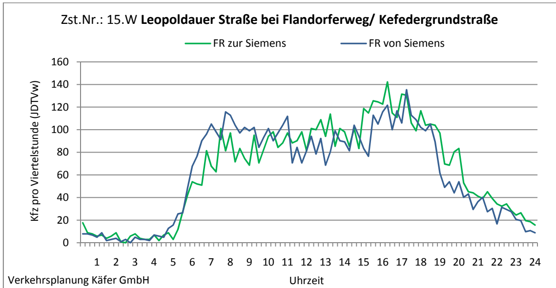
Abbildung 4-117: Tagesganglinien Leopoldauer Straße bei Flandorferweg/ Kefedergrundstraße (Zst. Nr.: 15.W)
