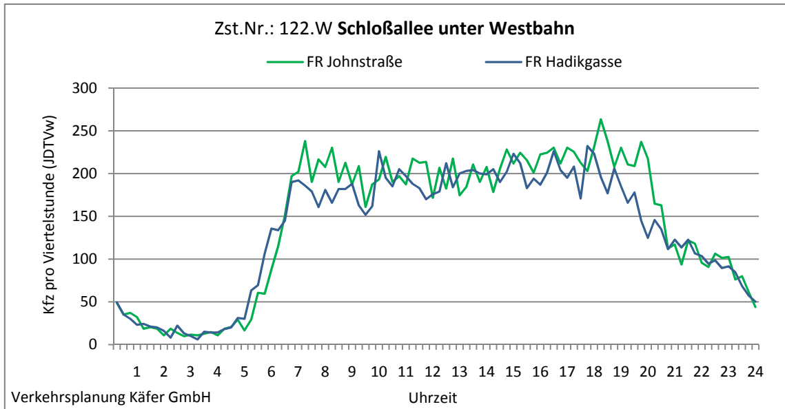
Abbildung 4-43: Tagesganglinien Schloßallee unter Westbahn (Zst. Nr.: 122.W)
