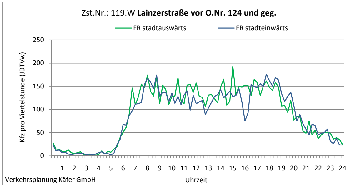
Abbildung 4-41: Tagesganglinien Lainzerstraße vor O.Nr. 124 und geg. (Zst. Nr.: 119.W)
