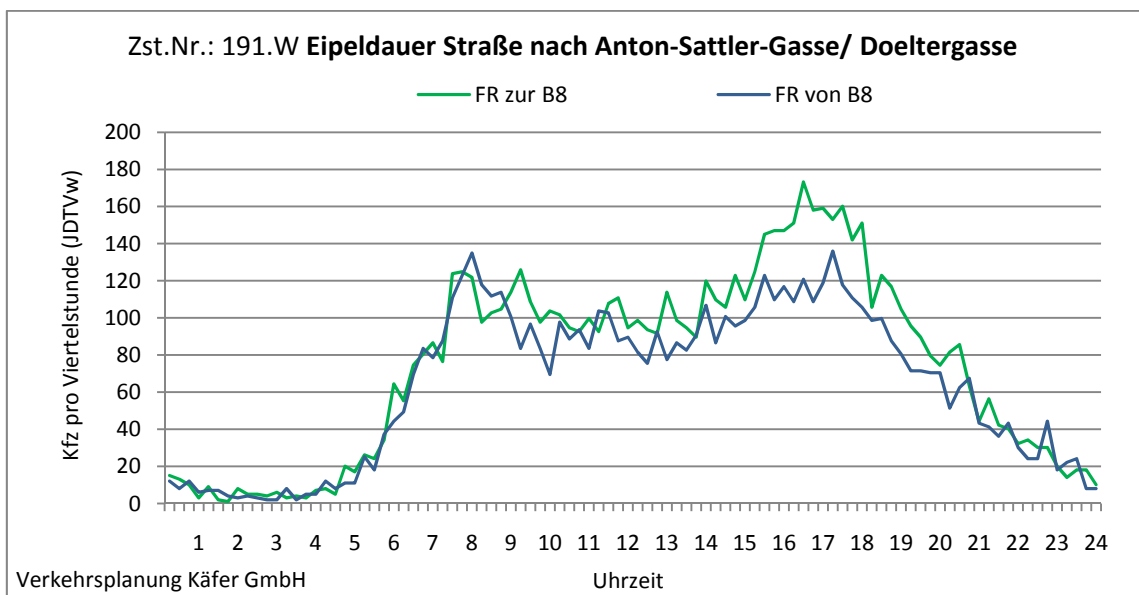
Abbildung 4-118: Tagesganglinien Eipeldauer Straße nach Anton-Sattler-Gasse/ Doeltergasse (Zst. Nr.: 191.W)
