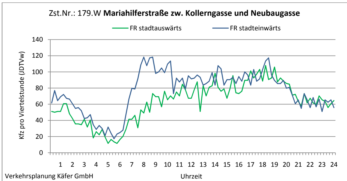
Abbildung 4-82: Tagesganglinien Mariahilferstraße zw. Kollerngasse und Neubaugasse (Zst. Nr.: 179.W)
