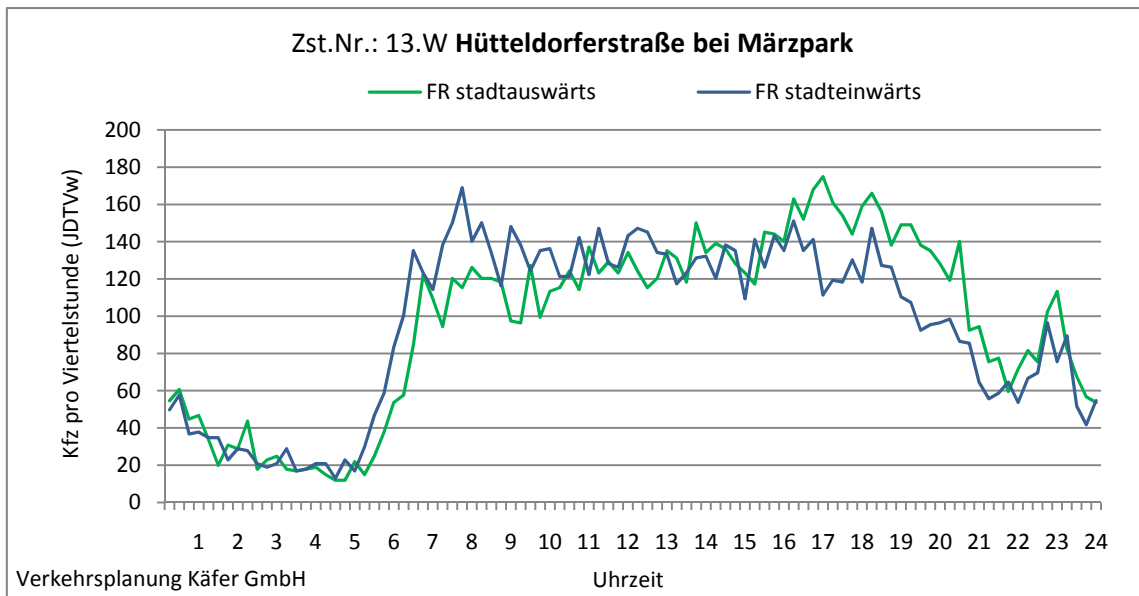
Abbildung 4-35: Tagesganglinien Hütteldorferstraße bei Märzpark (Zst. Nr.: 13.W)
