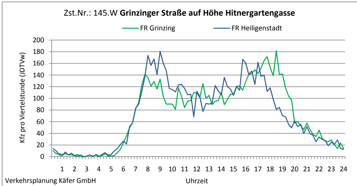
Abbildung 4-61: Tagesganglinien Grinzinger Straße auf Höhe Hitnergartengasse (Zst. Nr.: 145.W)
