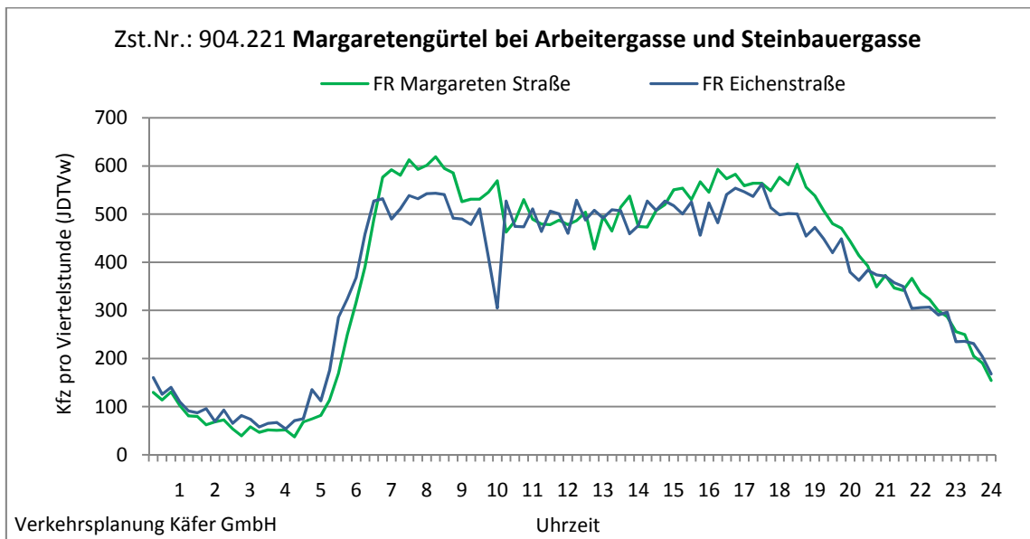
Abbildung 4-14: Tagesganglinien Margareteingürtel bei Arbeitergasse und Steinbauergasse (Zst. Nr.: 904.221)
