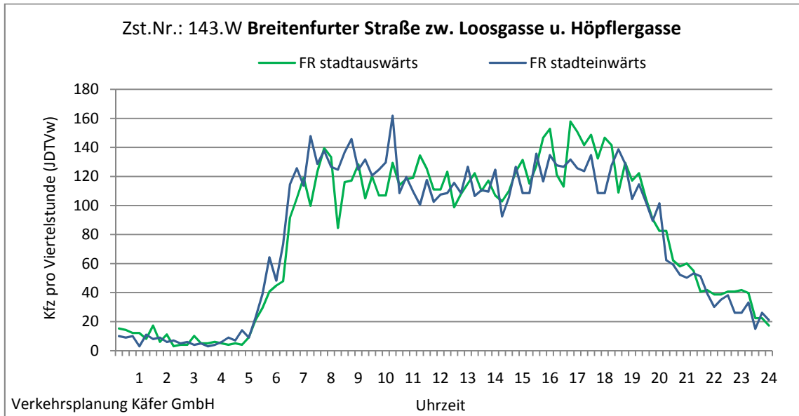
Abbildung 4-59: Tagesganglinien Breitenfurter Straße zw. Loosgasse u. Höpflergasse (Zst. Nr.: 143.W)
