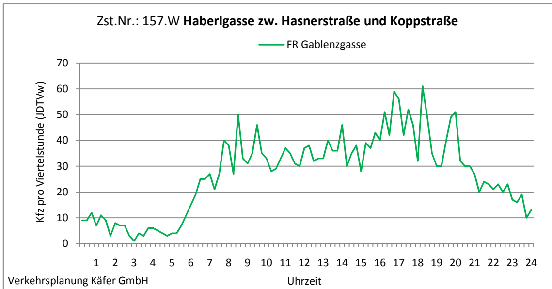
Abbildung 4-68: Tagesganglinie Haberlgasse zw. Hasnerstraße und Koppstraße (Zst. Nr.: 157.W)
