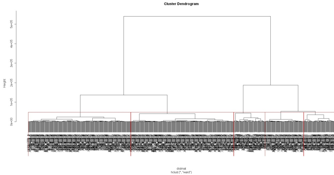
Abbildung 3-2: Clusteranalyse – Dendrogramm Fzg-Gruppe bis 6m
