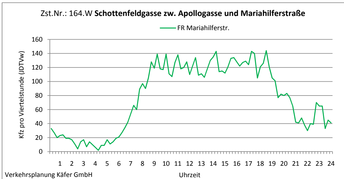
Abbildung 4-74: Tagesganglinie Schottenfeldgasse zw. Apollogasse und Mariahilferstraße (Zst. Nr.: 164.W)
