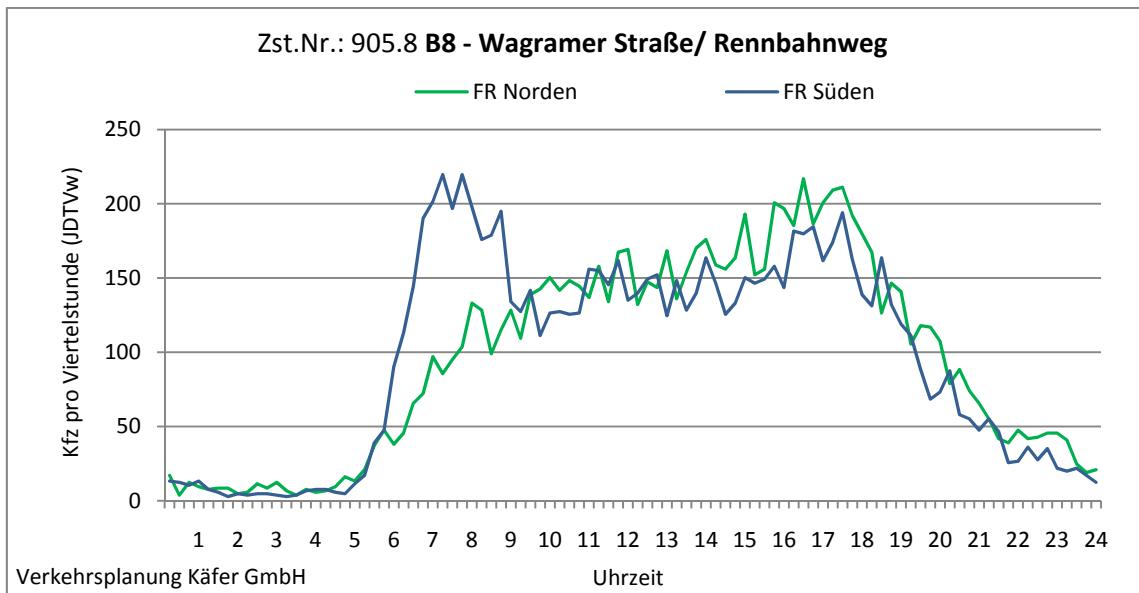
Abbildung 4-114: Tagesganglinien B8 Wagramer Straße/ Rennbahnweg (Zst. Nr.: 905.8)
