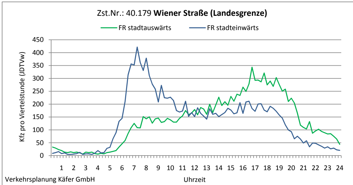
Abbildung 4-1: Tagesganglinien Wiener Straße (Zst. Nr.: 40.179)
