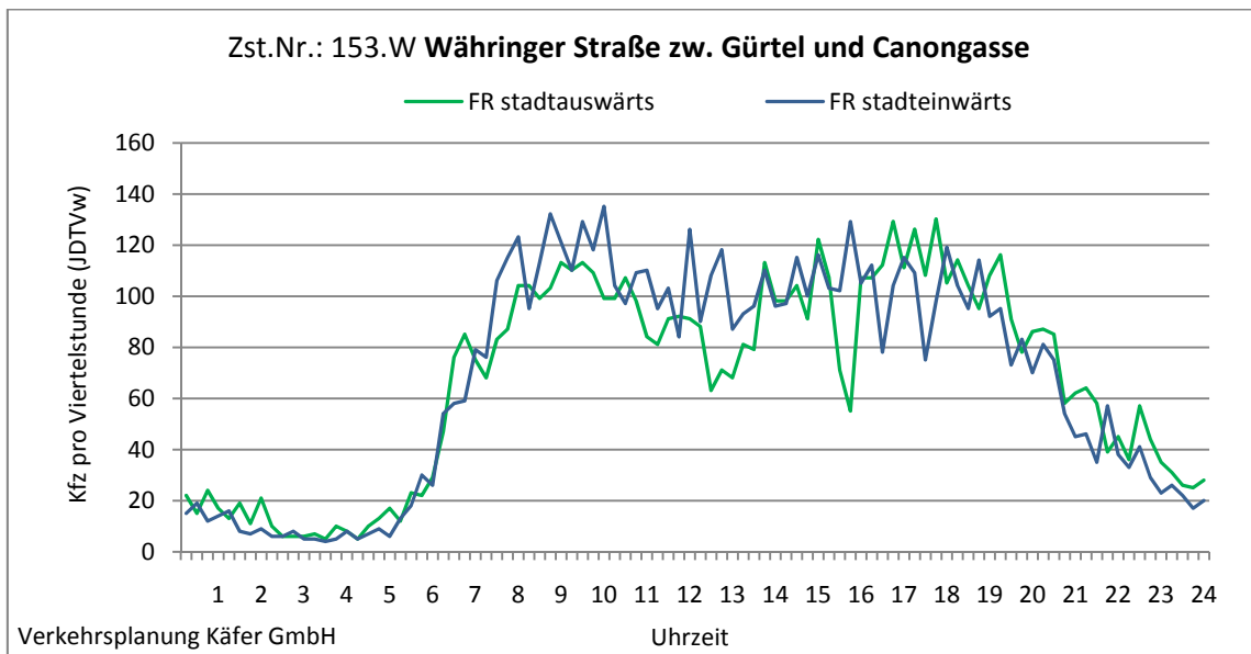
Abbildung 4-66: Tagesganglinien Währinger Straße zw. Gürtel und Canongasse (Zst. Nr.: 153.W)
