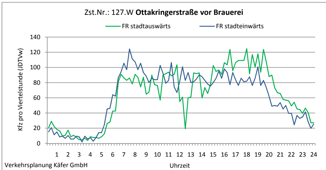
Abbildung 4-48: Tagesganglinien Ottakringerstraße vor Brauerei (Zst. Nr.: 127.W)
