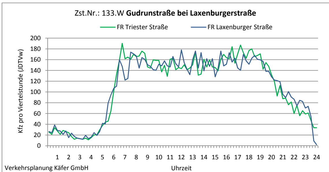
Abbildung 4-52: Tagesganglinien Gudrunstraße bei Laxenburgerstraße (Zst. Nr.: 133.W)
