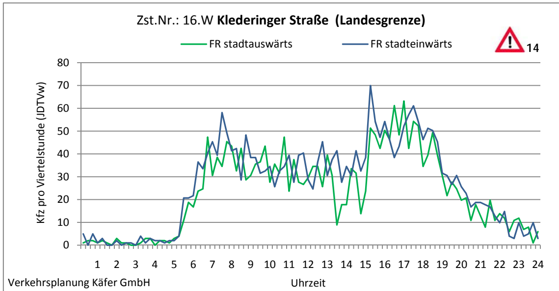
Abbildung 4-37: Tagesganglinien Klederinger Straße (Landesgrenze) (Zst. Nr.: 16.W)
