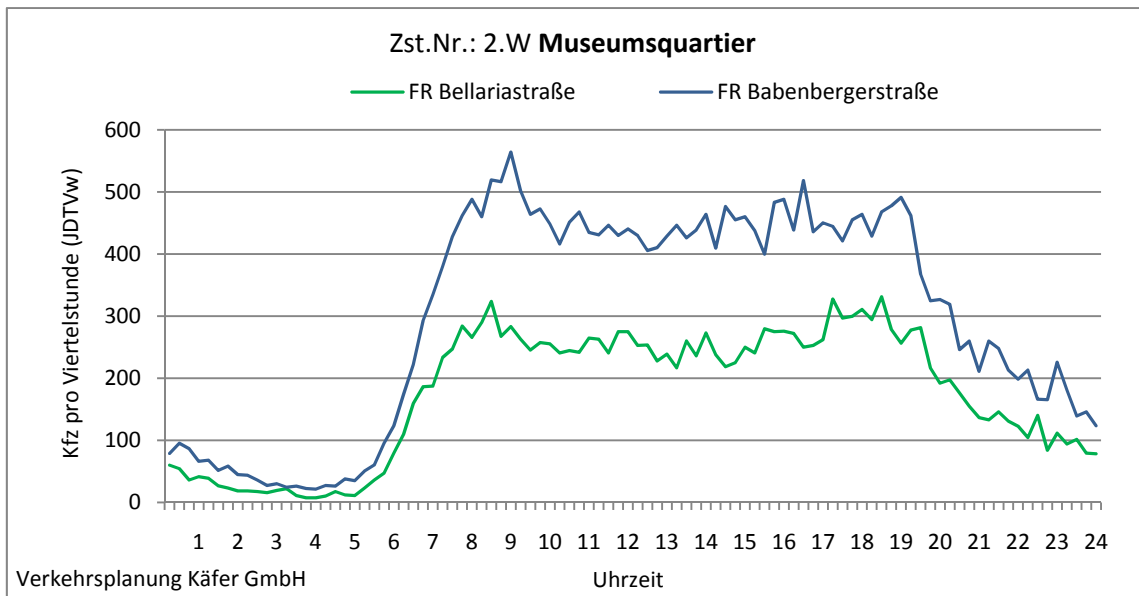
Abbildung 4-30: Tagesganglinien Museumsquartier (Zst. Nr.: 2.W)
