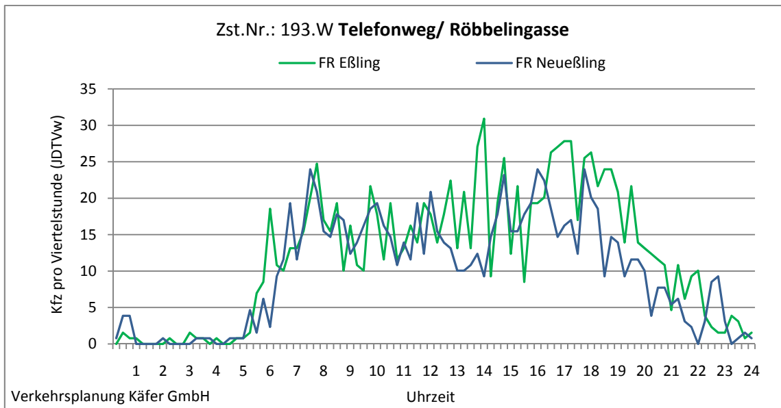
Abbildung 4-98: Tagesganglinien Telefonweg/ Röbbelingasse (Zst. Nr.: 193.W)
