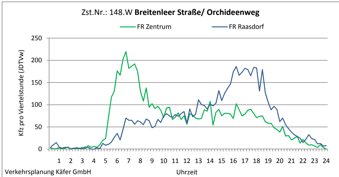
Abbildung 4-97: Tagesganglinien Breitenleer Straße/ Orchideenweg (Zst. Nr.: 148.W)
