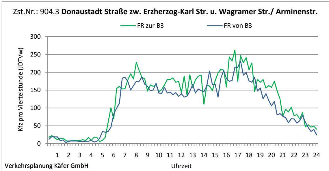
Abbildung 4-111: Tagesganglinien Donaustadt Straße zw. Erzherzog-Karl-Str. u. Wagramer Str./ Arminenstr. (Zst. Nr.: 904.3)
