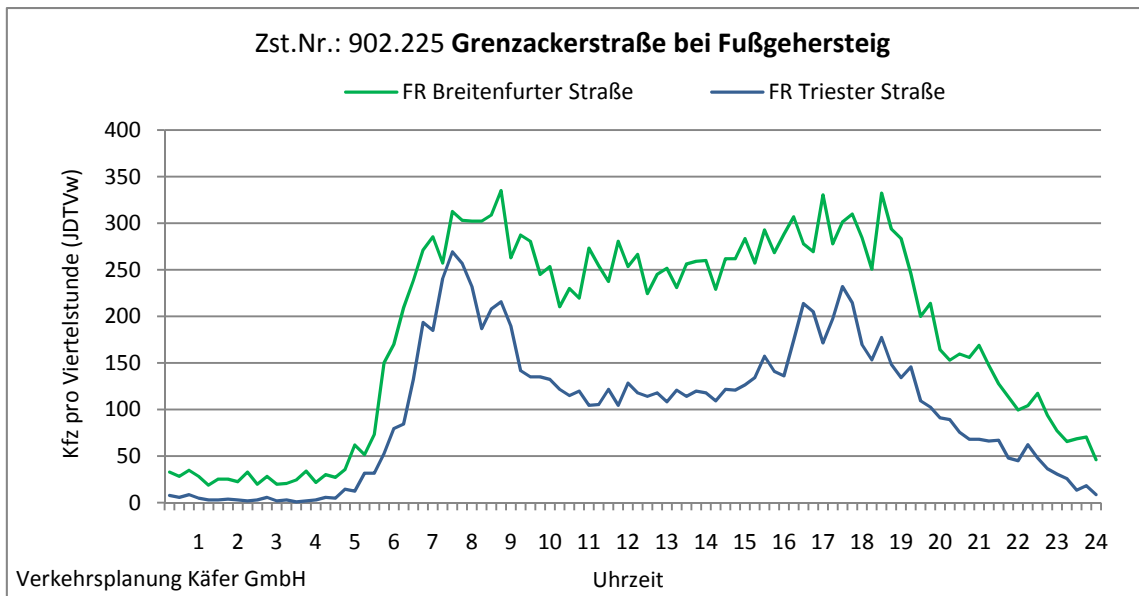
Abbildung 4-23: Tagesganglinien Grenzackerstraße bei Fußgehersteig (Zst. Nr.: 902.225)
