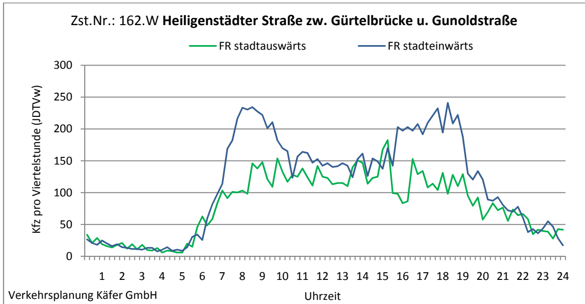
Abbildung 4-73: Tagesganglinien Heiligenstädter Straße zw. Gürtelbrücke u. Gunoldstraße (Zst. Nr.: 162.W)
