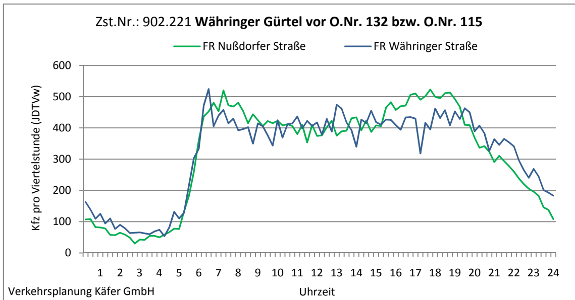
Abbildung 4-13: Tagesganglinien Währinger Gürtel vor O.Nr. 132 bzw. O.Nr. 115 (Zst. Nr.: 902.221)
