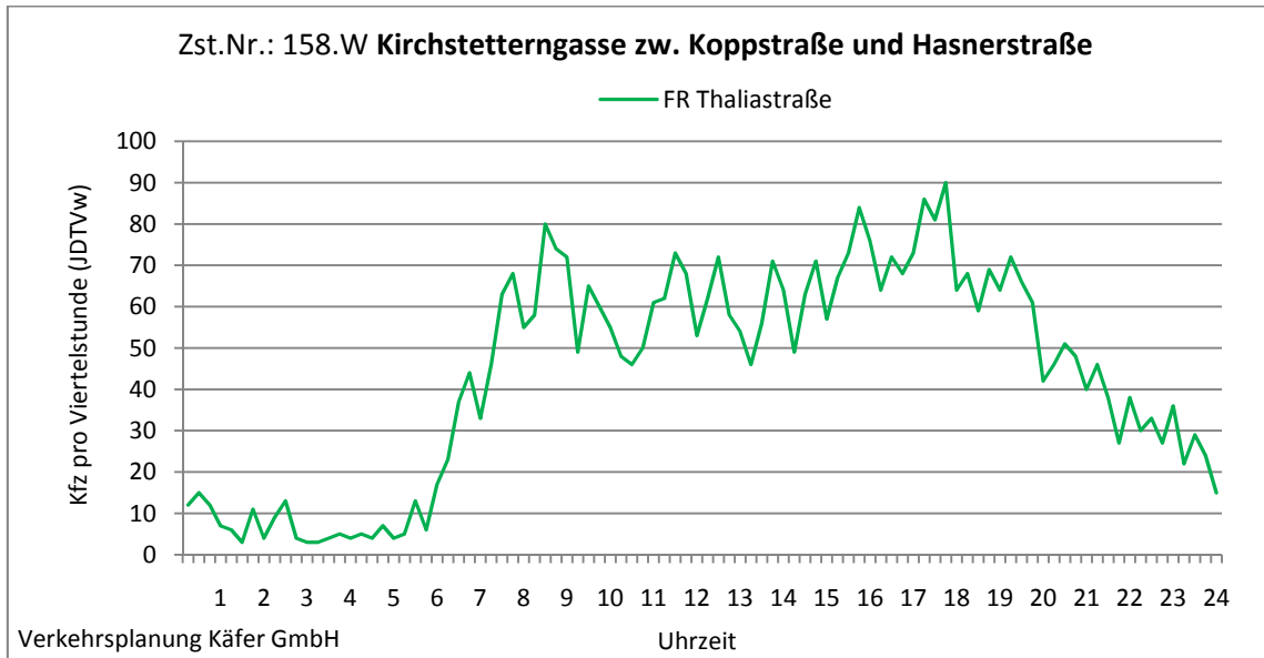
Abbildung 4-69: Tagesganglinie Kirchstetterngasse zw. Koppstraße und Hasnerstraße (Zst. Nr.: 158.W)
