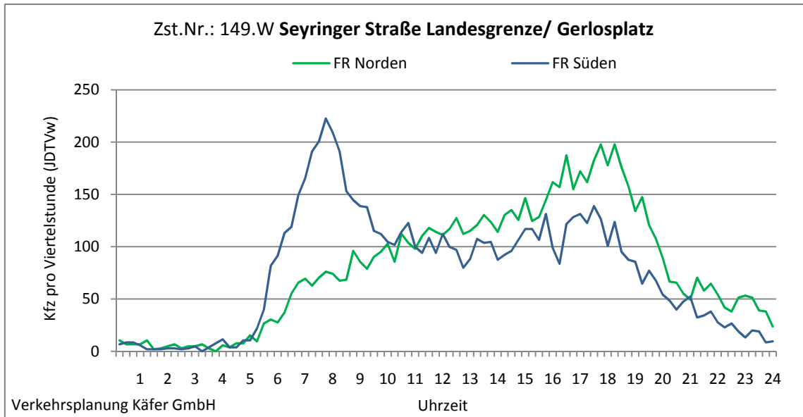
Abbildung 4-115: Tagesganglinien Seyringer Straße Landesgrenze/ Gerlosplatz (Zst. Nr.: 149.W)
