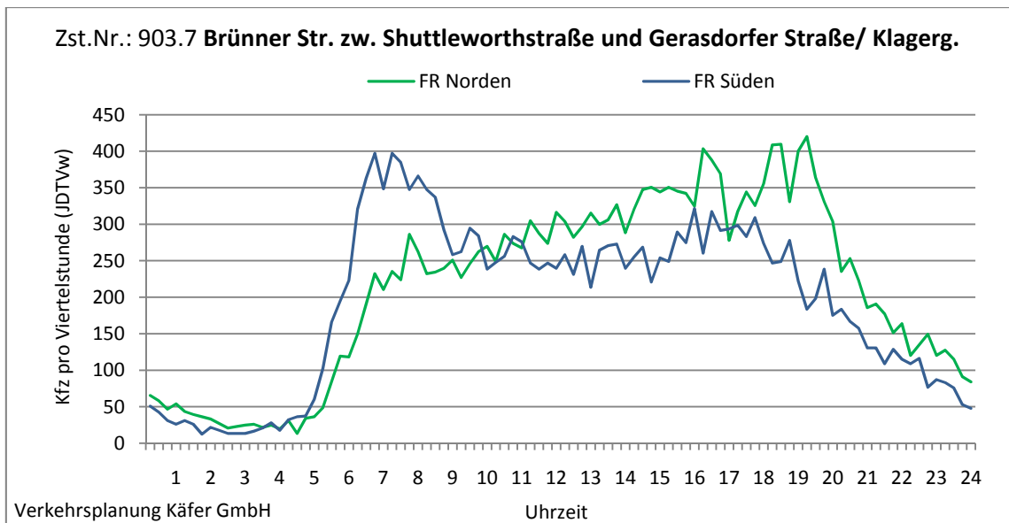
Abbildung 4-130: Tagesganglinien Brünner Str. zw. Shuttleworthstraße und Gerasdorfer Straße/ Klagerg. (Zst. Nr.: 903.7)
