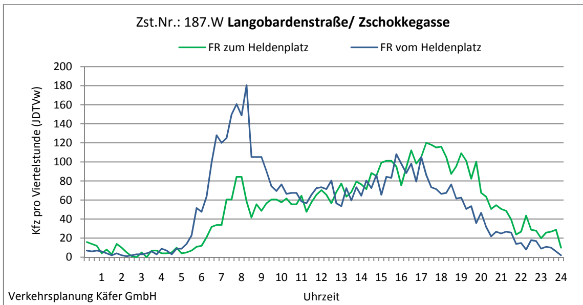
Abbildung 4-102: Tagesganglinien Langobardenstraße/ Zschokkegasse (Zst. Nr.: 187.W)
