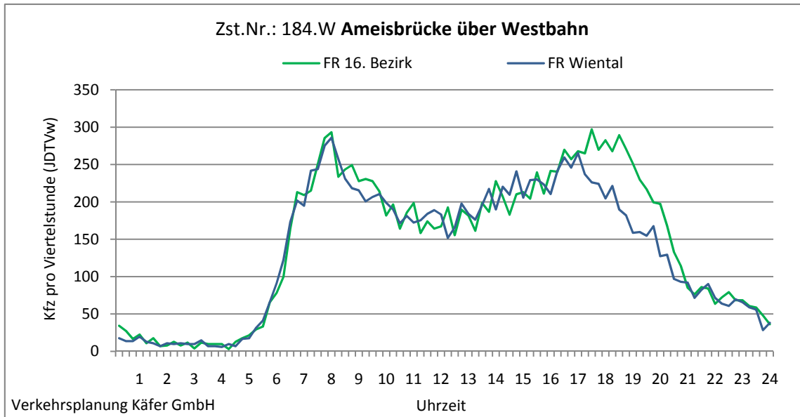
Abbildung 4-85: Tagesganglinien Ameisbrücke über Westbahn (Zst. Nr.: 184.W)
