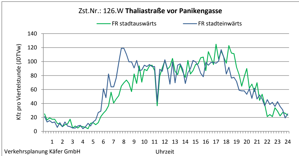
Abbildung 4-47: Tagesganglinien Thaliastraße vor Panikengasse (Zst. Nr.: 126.W)
