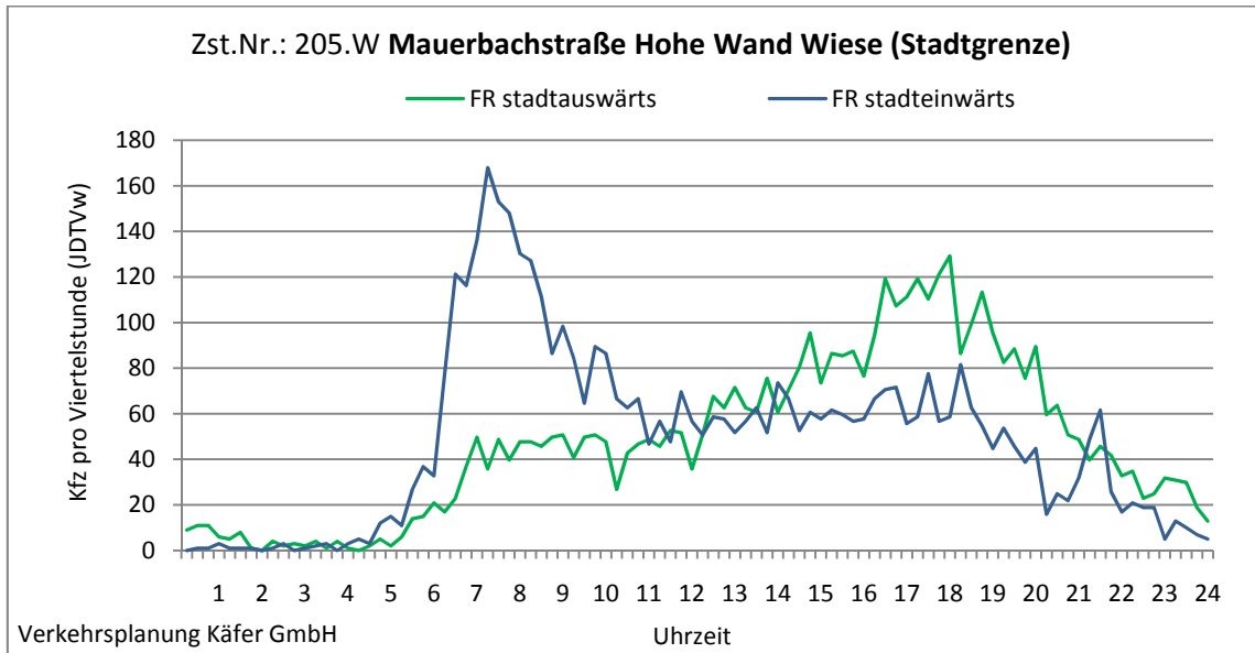
Abbildung 4-91: Tagesganglinien Mauerbachstraße Hohe Wand Wiese (Stadtgrenze) (Zst. Nr.: 205.W)
