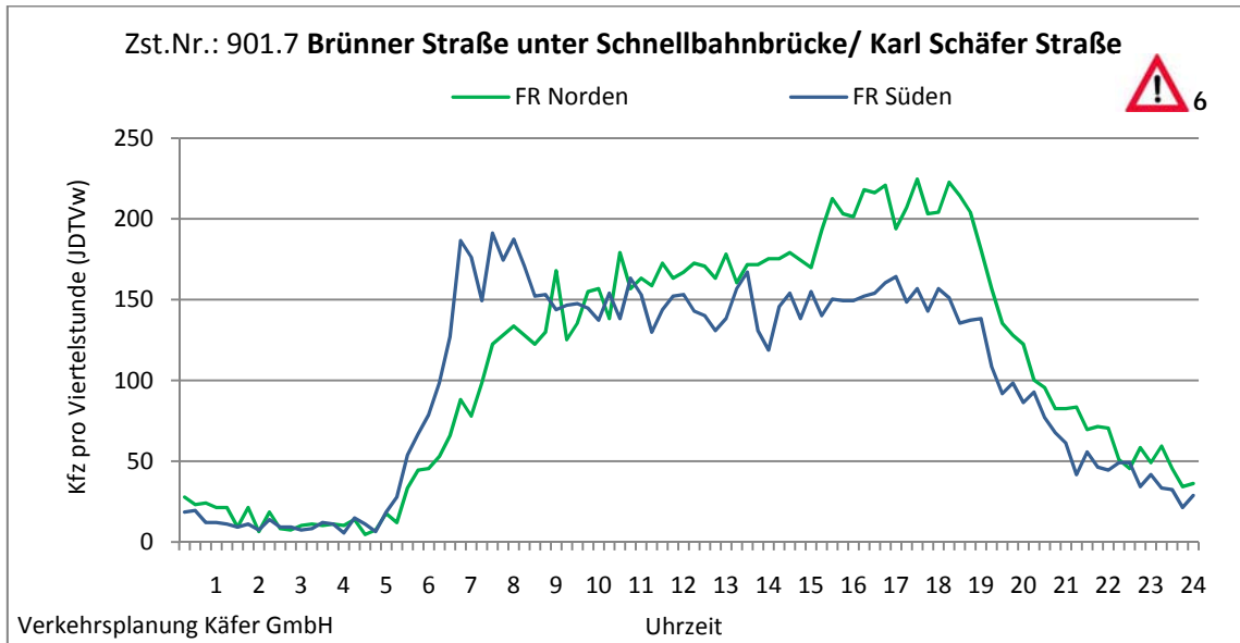
Abbildung 4-129: Tagesganglinien Brünner Straße unter Schnellbahnbrücke/ Karl Schäfer Straße (Zst. Nr.: 901.7)
