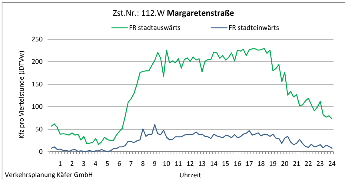
Abbildung 4-38: Tagesganglinien Margaretenstraße (Zst. Nr.: 112.W)
