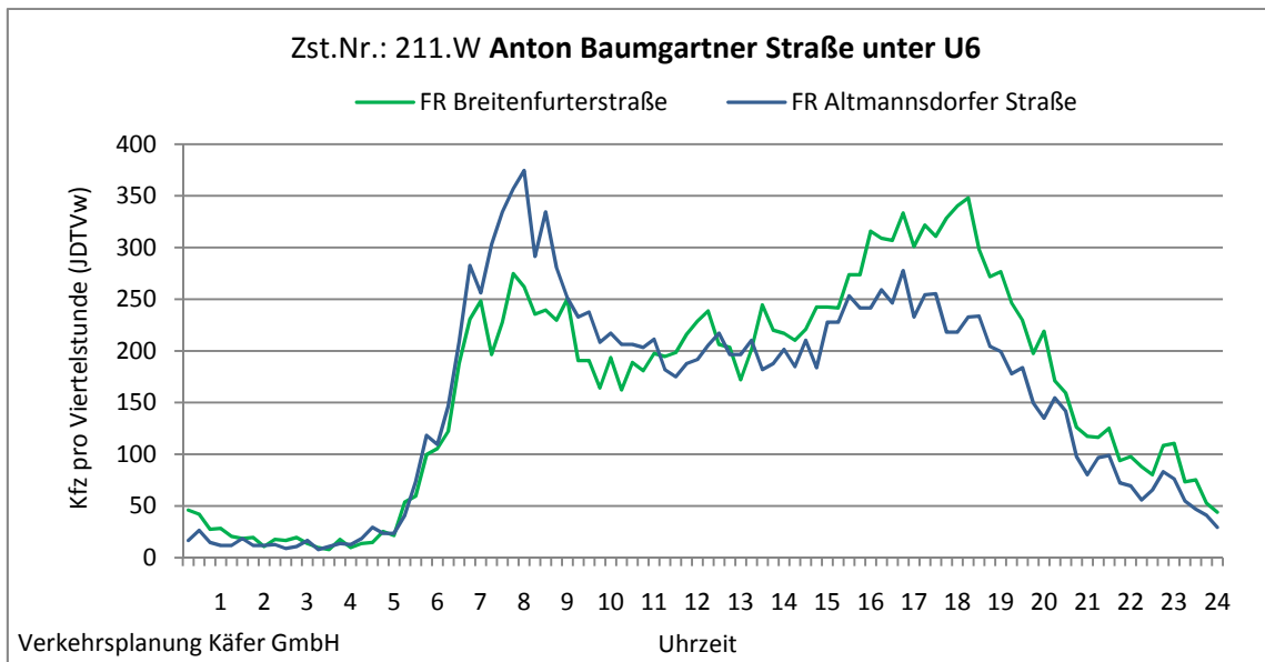
Abbildung 4-94: Tagesganglinien Anton Baumgartner Straße unter U6 (Zst. Nr.: 211.W)
