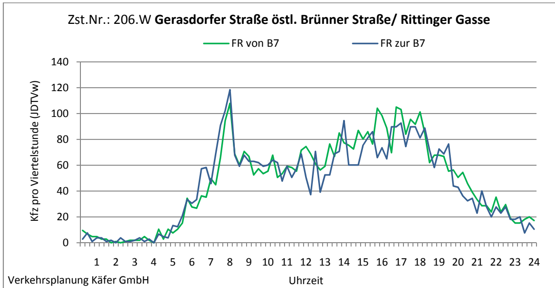
Abbildung 4-123: Tagesganglinien Gerasdorfer Straße östl. Brünner Straße/ Rittinger Gasse (Zst. Nr.: 206.W)
