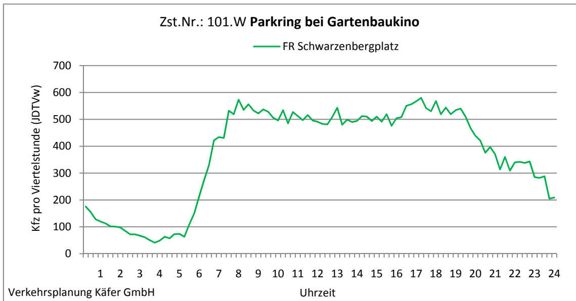
Abbildung 4-36: Tagesganglinie Parkring bei Gartenbaukino (Zst. Nr.: 101.W)
