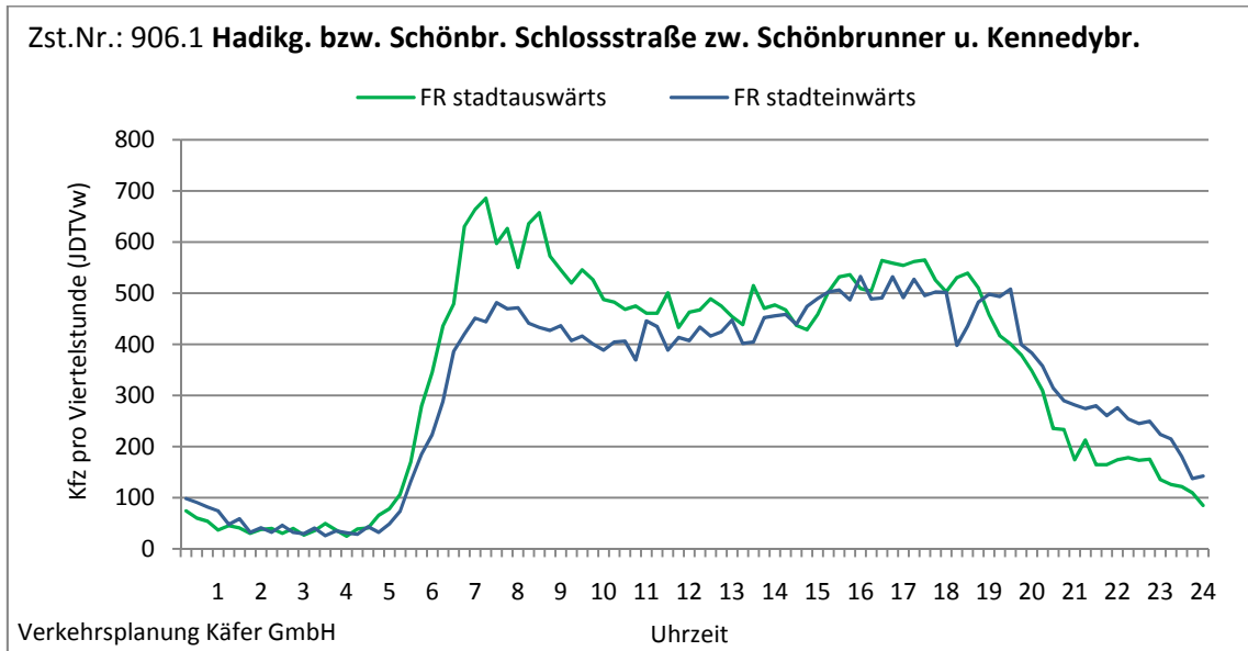
Abbildung 4-5: Tagesganglinien Hadikg. bzw. Schönbr. Schlosstraße zw. Schönbrunner u. Kennedybrücke (Zst. Nr.: 906.1)
