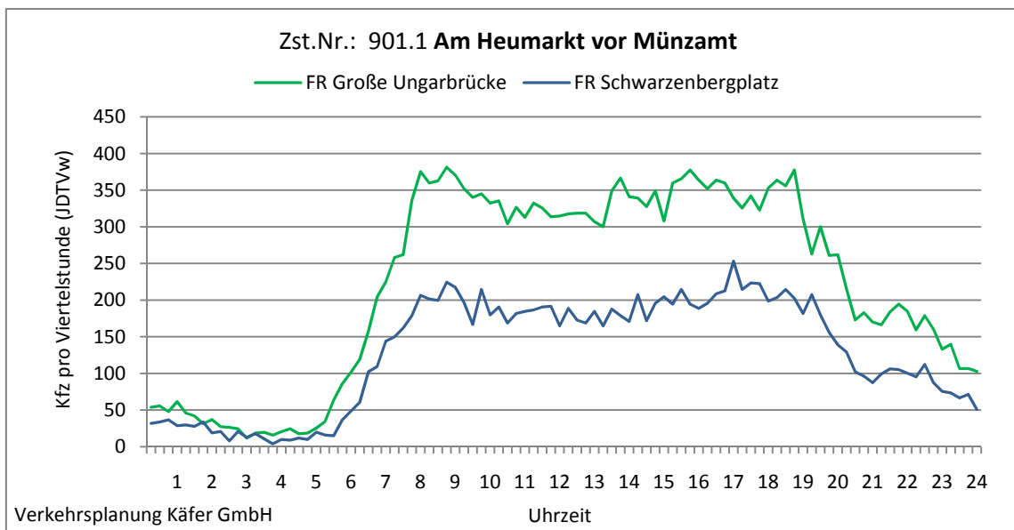
Abbildung 4-2: Tagesganglinien Am Heumarkt vor Münzamt (Zst. Nr.: 901.1)
