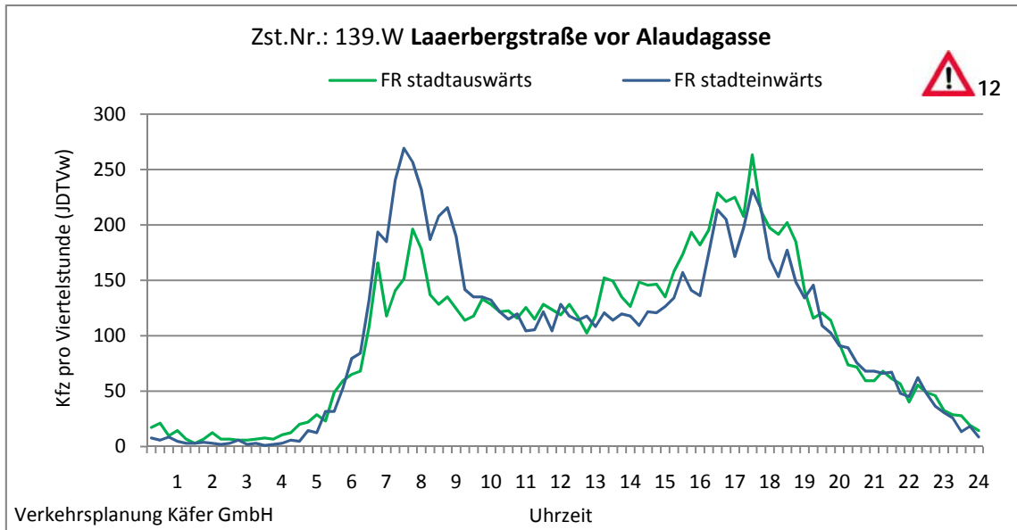
Abbildung 4-57: Tagesganglinien Laaerbergstraße vor Alaudagasse (Zst. Nr.: 139.W)
