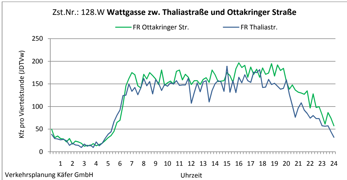
Abbildung 4-49: Tagesganglinien Wattgasse zw. Thaliastraße und Ottakringer Straße (Zst. Nr.: 128.W)
