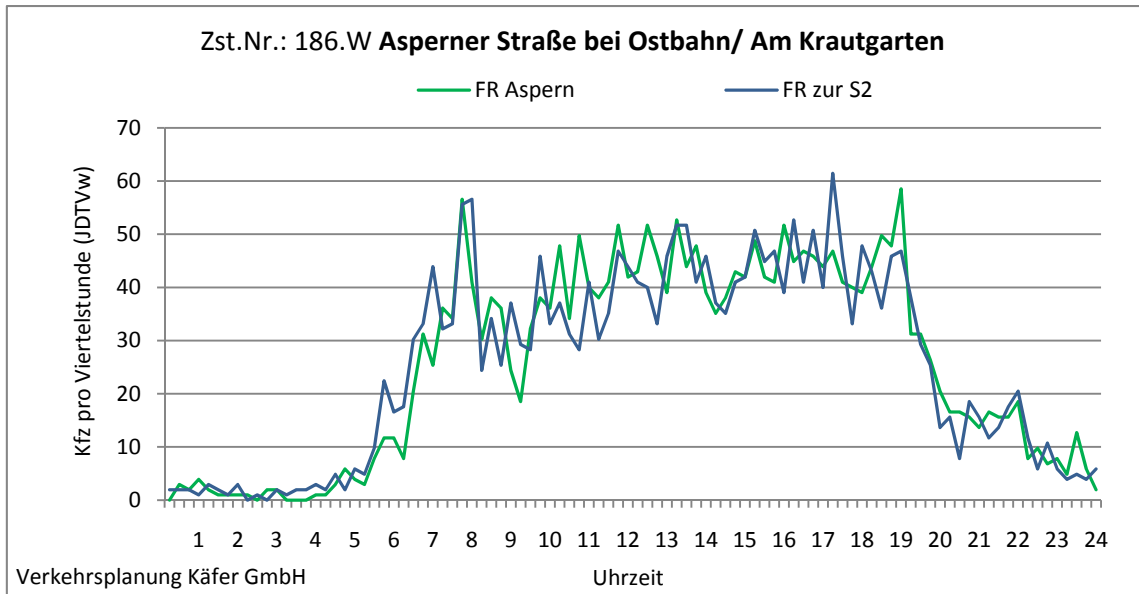
Abbildung 4-105: Tagesganglinien Aspener Straße bei Ostbahn/ Am Krautgarten (Zst. Nr.: 186.W)
